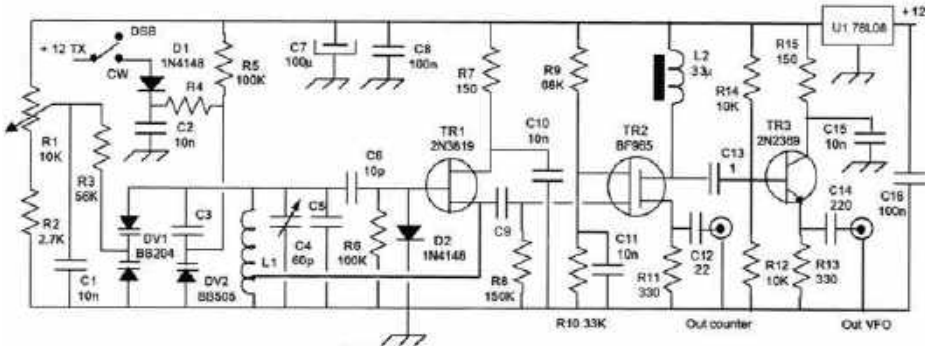
Rys. 3. Schemat ideowy układu VFO
