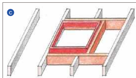
❶ Montaż okna dachowego na krokwiach (a), łatach (b), wymianach (c).
