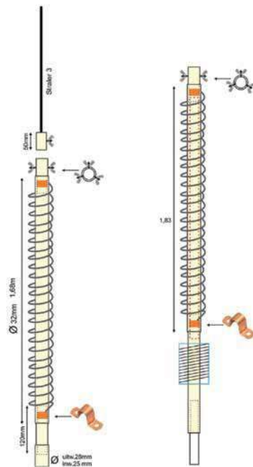
Rys. 6. Schemat anteny pionowej PA0EHC
