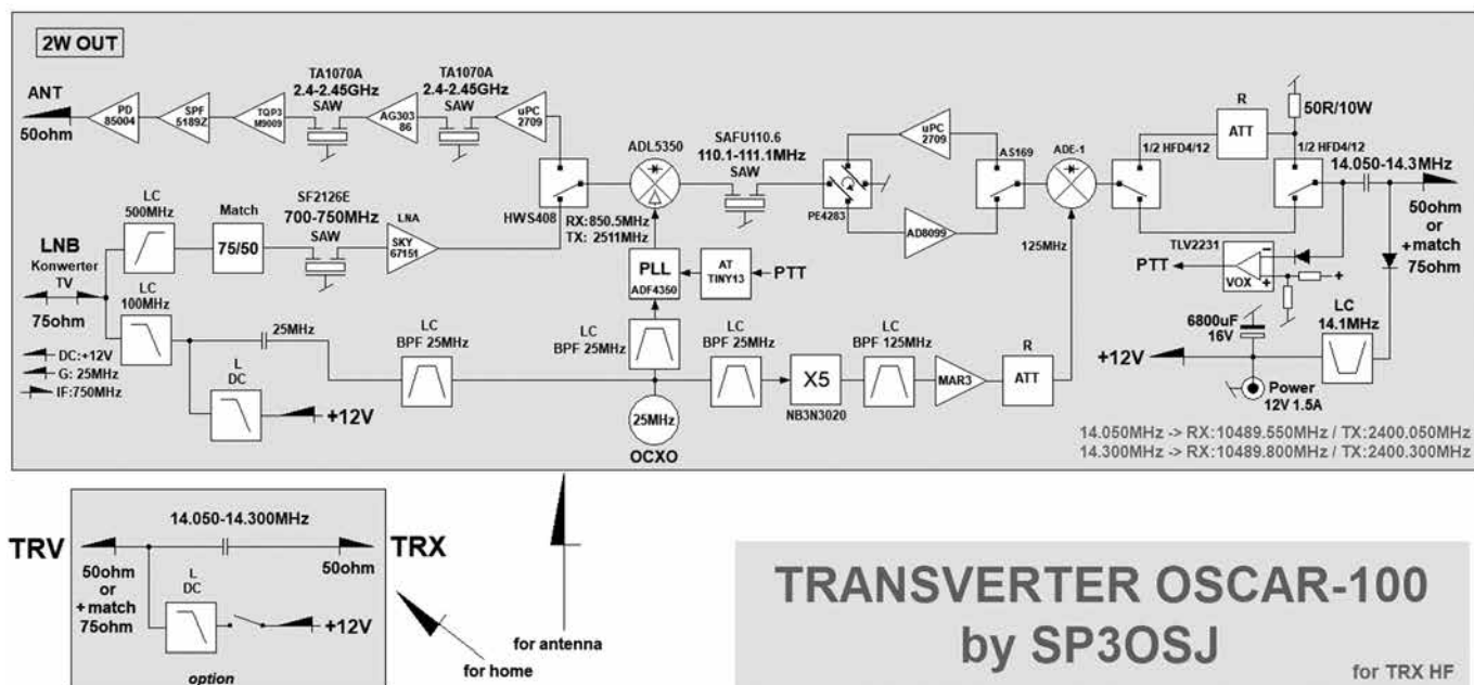
Rys. 1. Schemat blokowy transwertera
