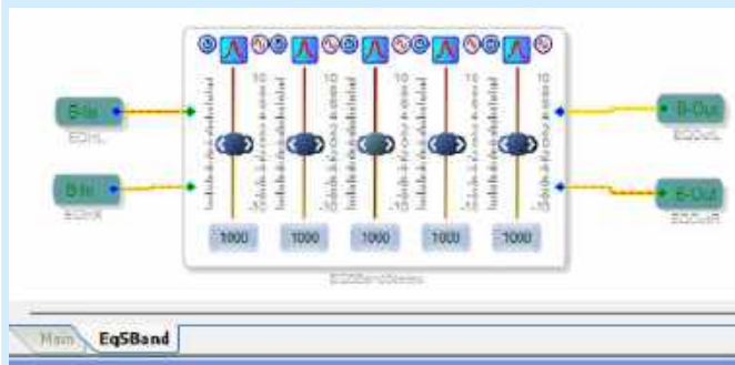
Rysunek 16. Przykładowy blok hierarchiczny EqsBand
