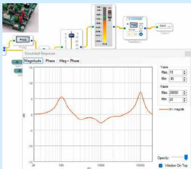
Rysunek 24. Przykładowa charakterystyka korekcji uzyskana z użyciem narzędzi Probe/Stimulus
