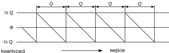
Rysunek 20. Okresowa funkcja błędów kwantyzacji idealnego kwantyzatora
