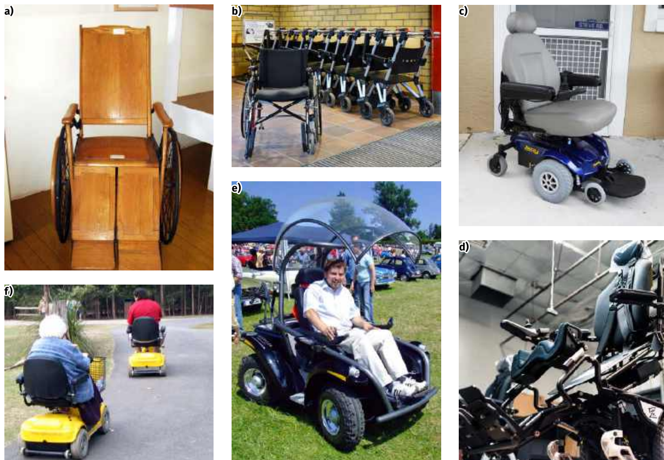
Fotografia 16. Wózki inwalidzkie różnych typów: drewniany wózek z początku XX wieku (a), współczesne wózki inwalidzkie: model składany i modele wsuwane jeden w drugi, w szwedzkim szpitalu (b), wózek elektryczny z napędem na przednie koła i siedziskiem „kapitańskim” (c), pionizator (d), wózek terenowy (e), skutery dla niepełnosprawnych (f). Źródło: Wikipedia.org
