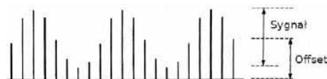
Rysunek 3. Impulsy na wyjściu idealnego przetwornika cyfrowo-analogowego
