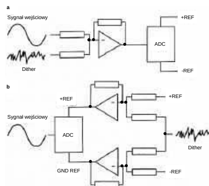
Rysunek 22. a) dither jest liniowo dodawany do analogowego sygnału wejściowego, b) dither jest dodawany do napięć odniesienia kwantyzatora
