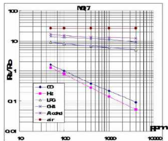
Rysunek 4. Typowa czułość czujnika MQ-7 na różne gazy [3]
