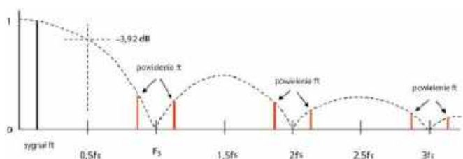
Rysunek 8. Charakterystyka częstotliwościowa sygnału schodkowego z wyjścia przetwornika
