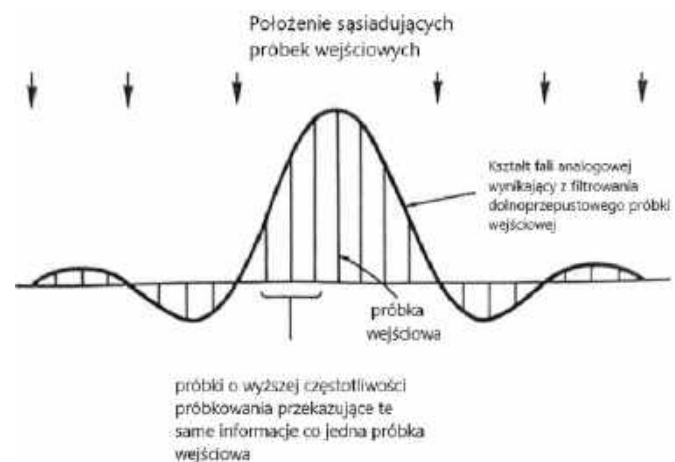
Rysunek 17. Idea działania interpolatora
