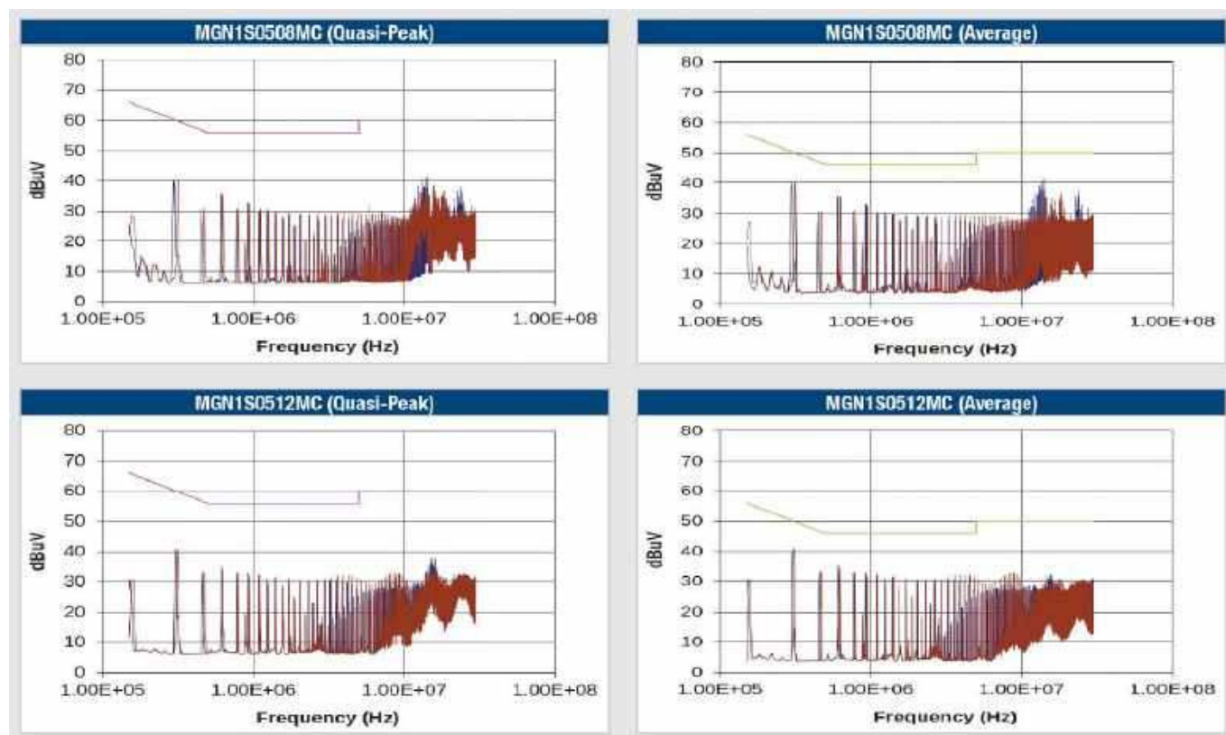
Rysunek 1. Wyniki badań w zakresie emisji zaburzeń EMI dla dwóch modeli przetwornic z serii MGN1 ( https://t.ly/nTCeC )
