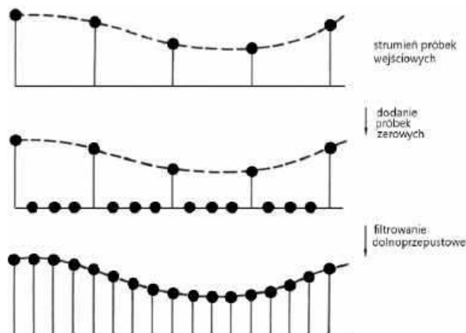
Rysunek 16. Idea działania filtra interpolatora
