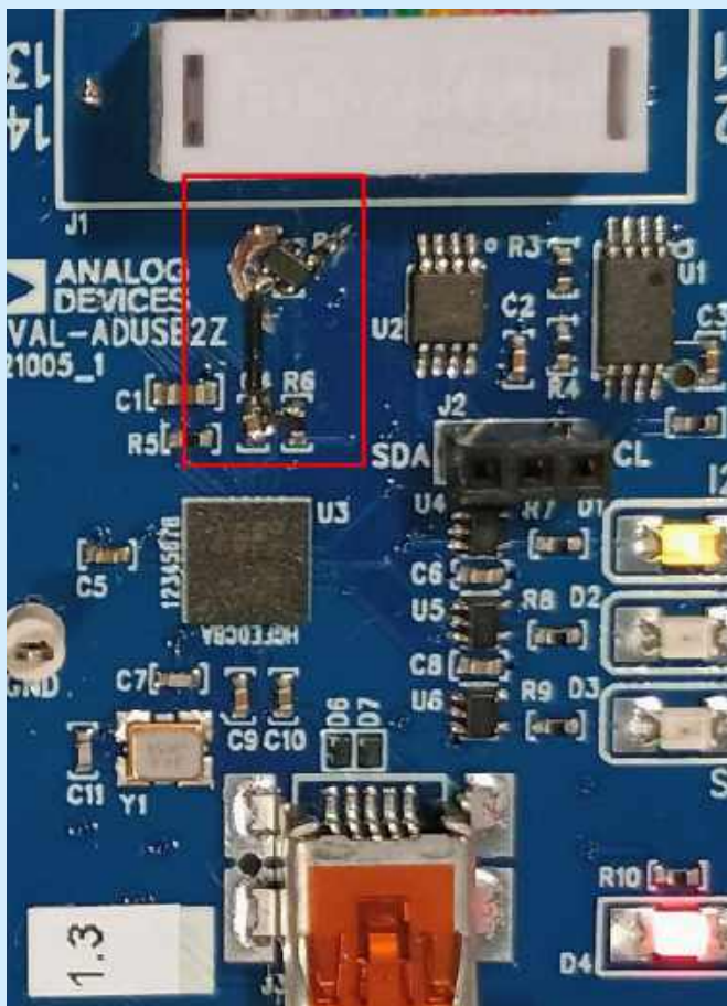
Fotografia 2. Zmodyfikowany programator USBi
