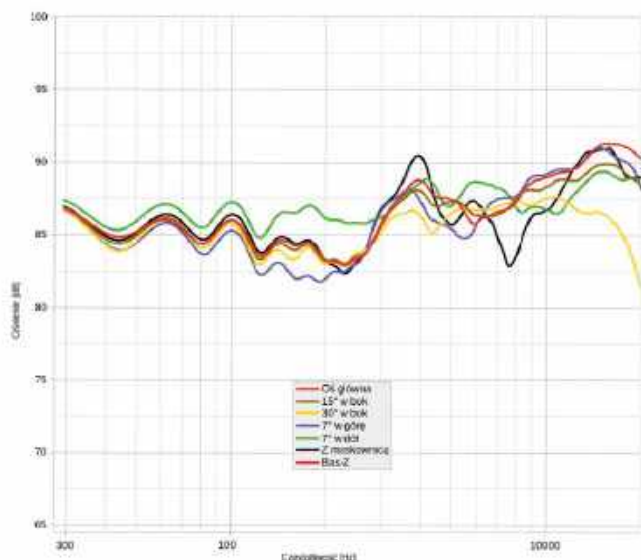
Rysunek 5. Charakterystyki wolno stojącego, dwupółdrożnego (abstrahując od wstęgowego superwysokotonowego) zespołu głośnikowego (Dali Rubikore 6, test w „AUDIO” 3/2025), w zakresie 300 Hz...20 kHz, zmierzone metodą MLS z odległości 1,5 m, pod różnymi kątami w płaszczyźnie poziomej i pionowej. Sytuacja jest dość znamienna dla układów dwupółdrożnych, gdzie w zakresie średnionotowym, znowu na skutek przesunięć fazowych, tym razem między przetwornikiem (nominalnie) niskotonowym a głośnikiem nisko-średnionotowym charakterystyka obniża się wraz z „oddalaniem” od niskotonowego (a więc pod kątem +7°, charakterystyka niebieska) i rośnie wraz ze zbliżaniem do niego (–7°, charakterystyka zielona). Na osi głównej (wyprowadzonej na osi głośnika wysokotonowego, na wysokości 90 cm) charakterystyka ma lżejsze osłabienie. Takim układowi głośników i filtrów dobrze posłużyłoby pochylenie obudowy do tyłu (a dokładnie – przedniej ścianki, co jednak wcale nie jest uniwersalnym sposobem na lepsze zestrojenie, jak sądzą niektórzy). Typowe dla konstrukcji firmy Dali jest wyeksponowanie wysokich tonów (na osi głównej), które z powodu „naturalnych” właściwości skupiania promieniowania musi ustępować na innych osiach, dlatego sam producent rekomenduje, aby kolumny ustawiać osiami głównymi biegnącymi daleko od miejsca odsłuchowego, nawet równolegle, a wtedy słuchacz znajdzie się na osi ok. 30° – czyli będzie słyszał charakterystykę żółtą, która biegnie najrówniej aż do 15 kHz. W pewnym sensie to zaplanowana przez producenta oś główna, a nie standardowa oś wyprowadzona na wprost kolumny
