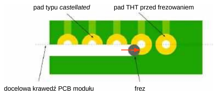
Rysunek 9. Proces wytwarzania padów typu castellated
