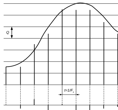
Rysunek 21. Powstawanie impulsów błędów kwantyzacji
