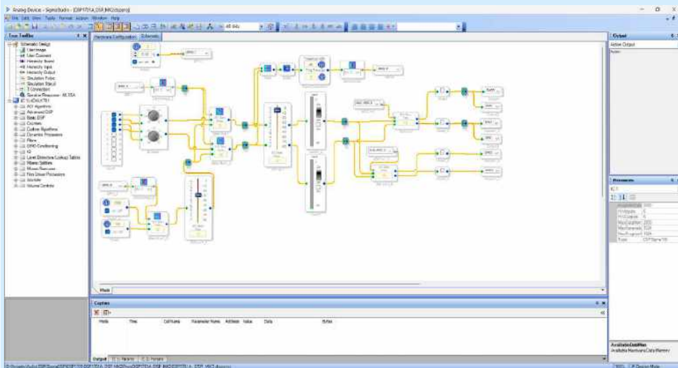
Rysunek 1. Oprogramowanie SigmaStudio
