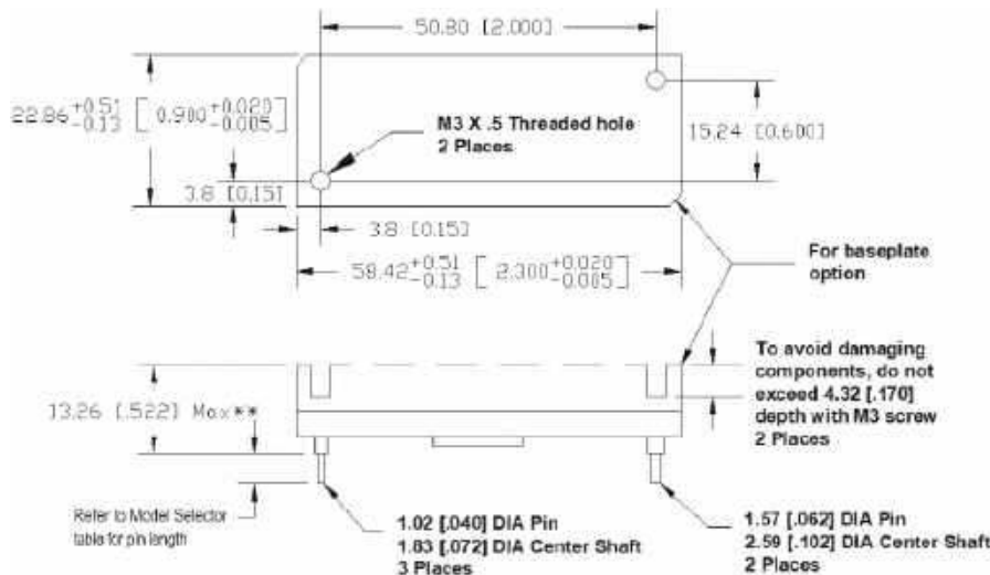
Rysunek 2. Wymiary miniaturowej przetwornicy z fotografii 3 ( https://t.ly/P9gzB )
