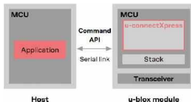
Rysunek 4. Przykład architektury systemu opartego na module wyposażonym w firmowe oprogramowanie wbudowane – moduł u-blox z wgranym pakietem u-connectXpress ( https://t.ly/CFx_k )
