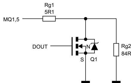
Rysunek 7. Modyfikacja modułu modMQ-7
