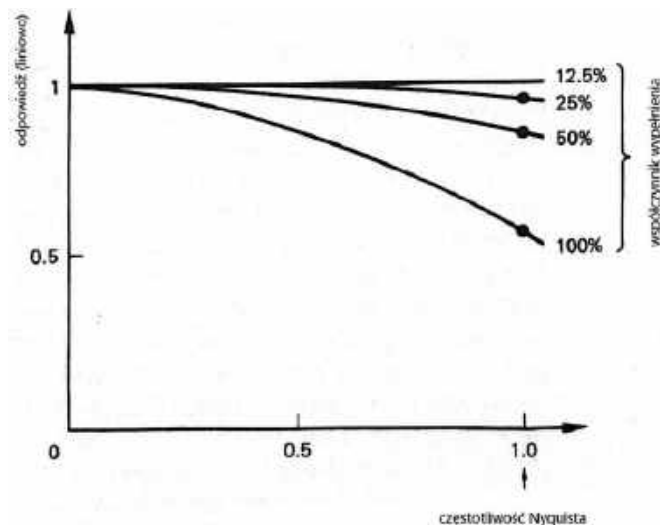
Rysunek 10. Charakterystyki amplitudowo-częstotliwościowe przy różnych wartościach apertur
