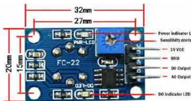
Rysunek 5. Moduł modMQ-7 [6]
