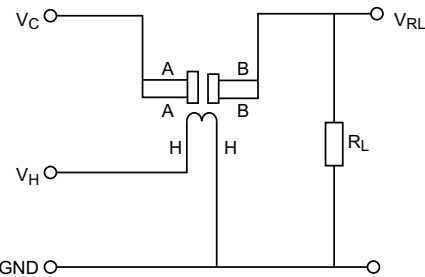
Rysunek 2. Standardowy układ pracy czujnika MQ-7 [4]
