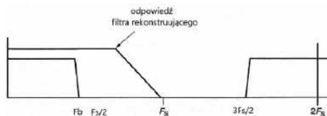
Rysunek 12. Odpowiedź częstotliwościowa filtra rekonstruującego przy nadpróbkowaniu 2- F_s
