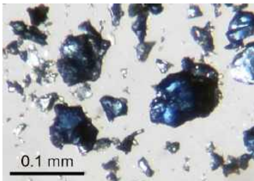
6. Kryształy ringwoodytu
