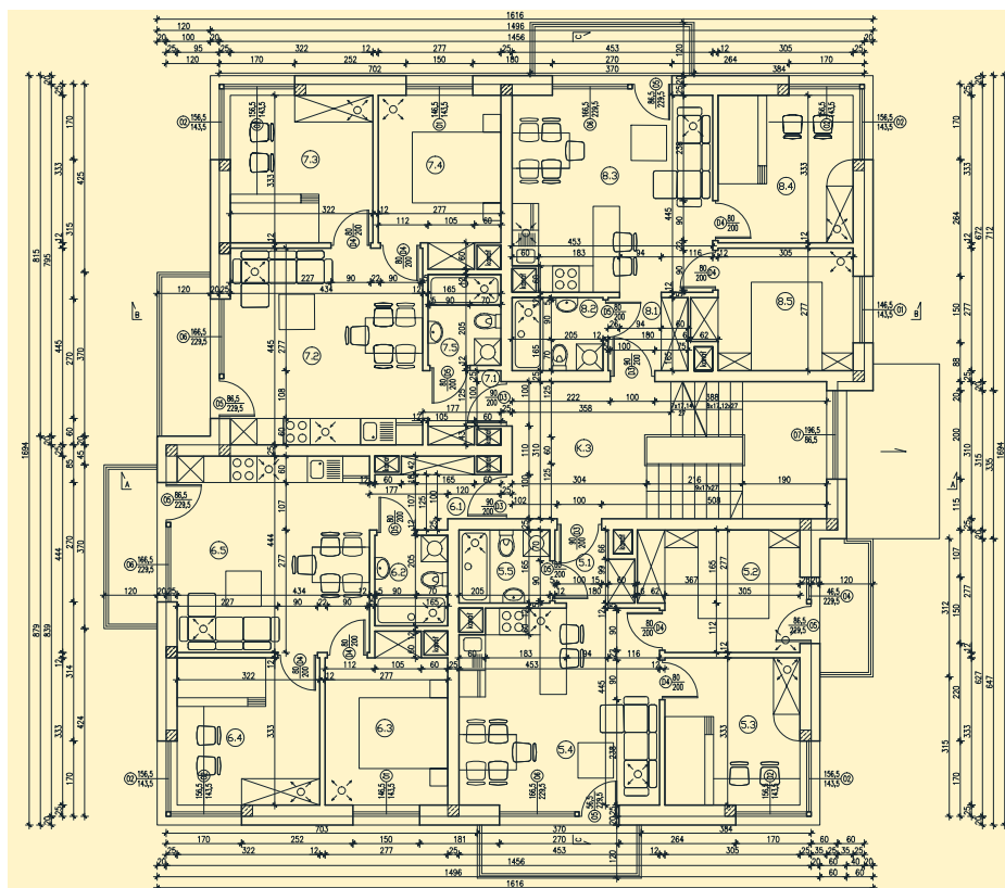
Rzut 1 piętra
