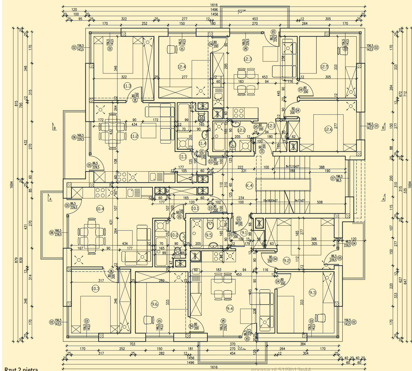
Rzut 2 piętra
