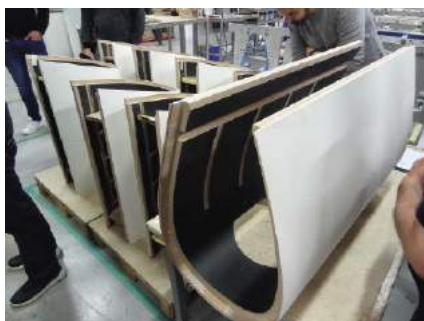
Skorupa zewnętrzna dopiero po uformowaniu jest dokładnie wycinana i frezowana.
