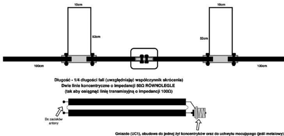
Rys. 6. Szkic budowy anteny 3 \times 1/2 fali
