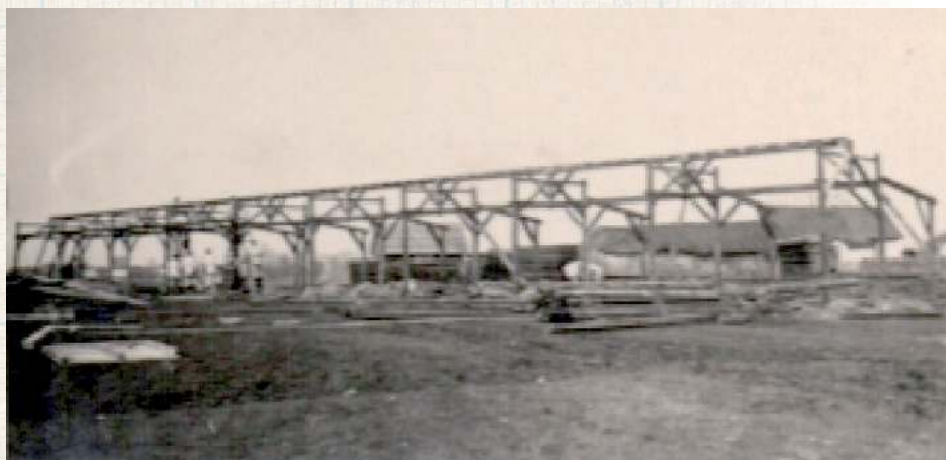
Konstrukcja szkieletu baraku mieszkalnego. Nie wiemy, czy budynek się zachował
