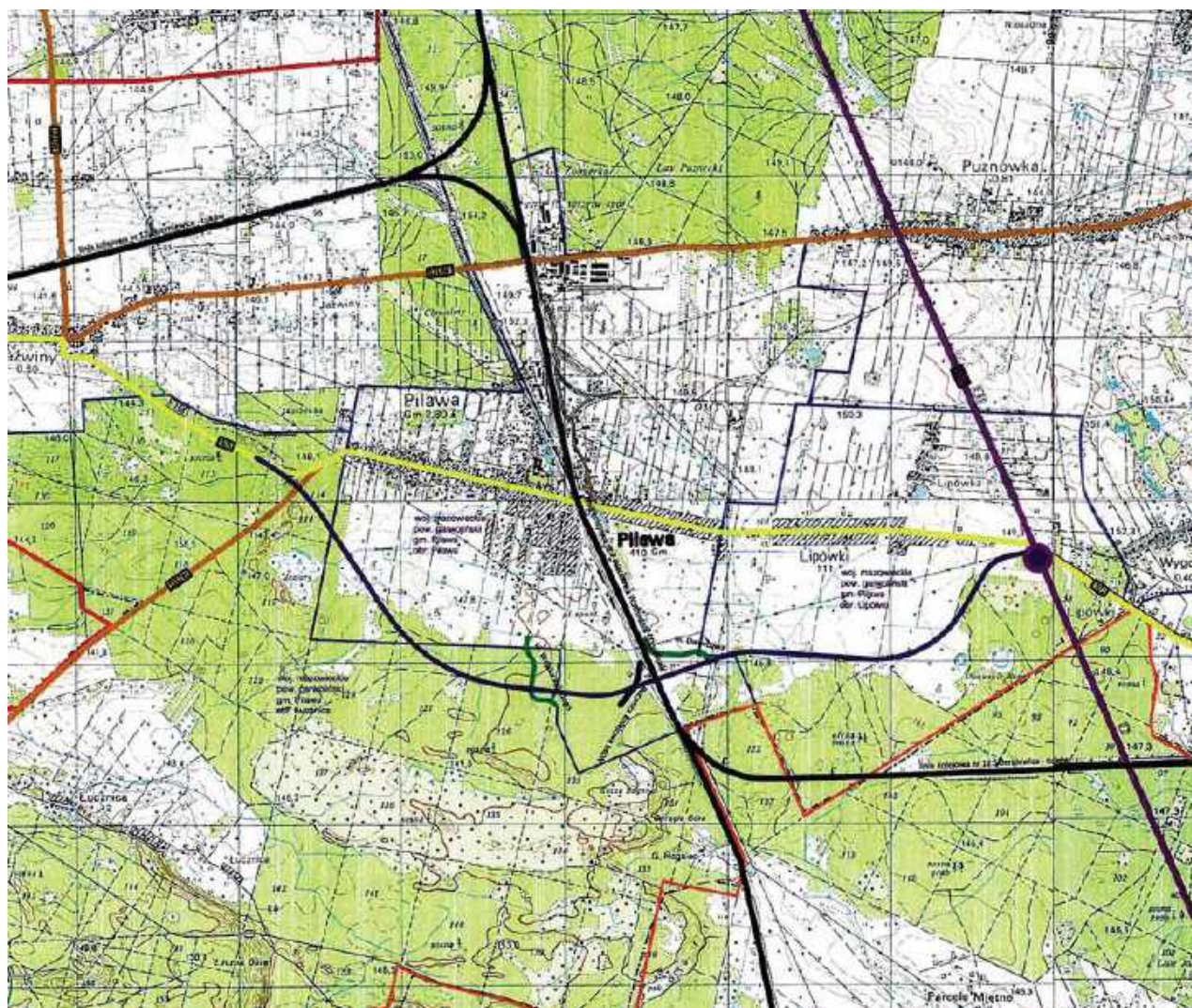
Projekt techniczny obwodnicy Pilawy z 2023 r.
