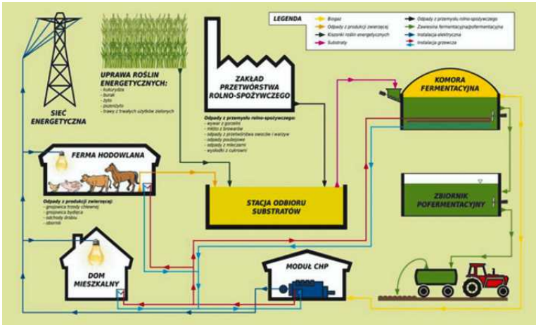
Schemat biogazowni rolniczej
