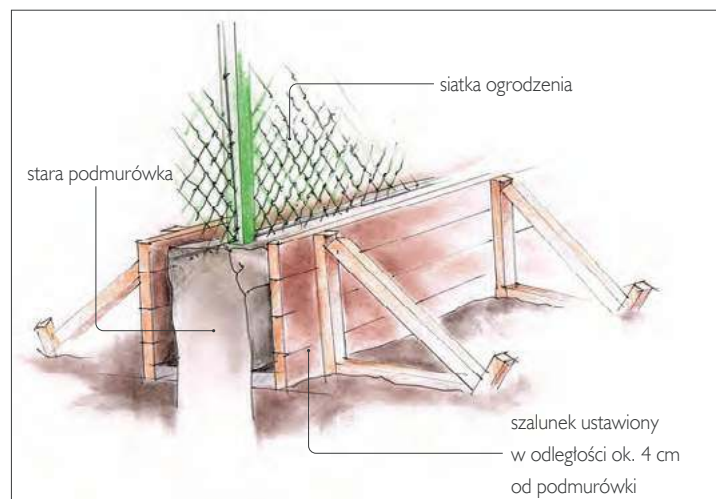
❶ Jednym ze sposobów naprawy ogrodzenia jest wylanie nowej osłony podmurówki w szalunku.
