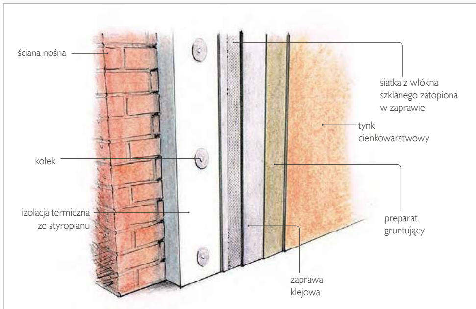
🔑 Ściana ocieplona metodą lekką mokrą.
