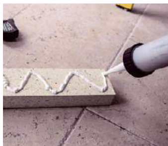
➊ Aplikacja kleju polimerowego na profil bazowy.
