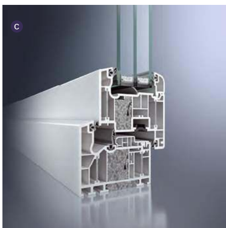
❶ Trzy różne profile: drewniany o głębokości 92 mm, z pakietem trzyszybowym, U_w 0,84 W/(m 2 ·K) (a MS WIĘCEJ NIŻ OKNA), 6-komorowy PVC o głębokości 82 mm, z pakietem trzyszybowym, U_w 0,77 W/(m 2 ·K) (b VETREX), 7-komorowy PVC z wzmocnieniami z aluminium, o głębokości 82 mm, przeznaczony do domów pasywnych, U_w od 0,64 W/(m 2 ·K) (c SCHÜCO).
