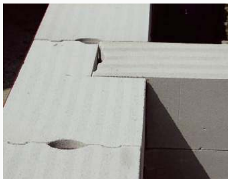
❗ Właściwe przemurzenie ścian to podstawa utworzenia stabilnej i wytrzymałej przegrody. T. RYBARCZYK
