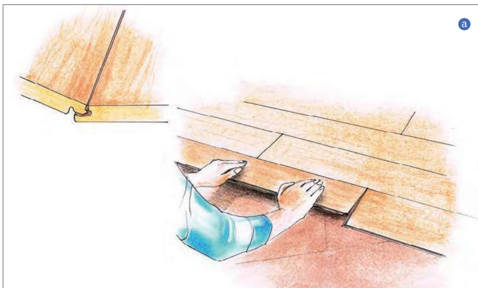
a Panele układamy wpustem (wystającą dolną częścią zamka) w stronę kolejnych rzędów (a) . Odstępy dylatacyjne na obwodzie posadzki uzyskamy poprzez wstawienie klinów (b) .
