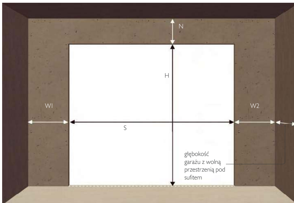
📏 Ważne wymiary otworu wjazdowego: S – szerokość, H – wysokość, N – wysokość nadproża, W1 i W2 – szerokość węgarków.
