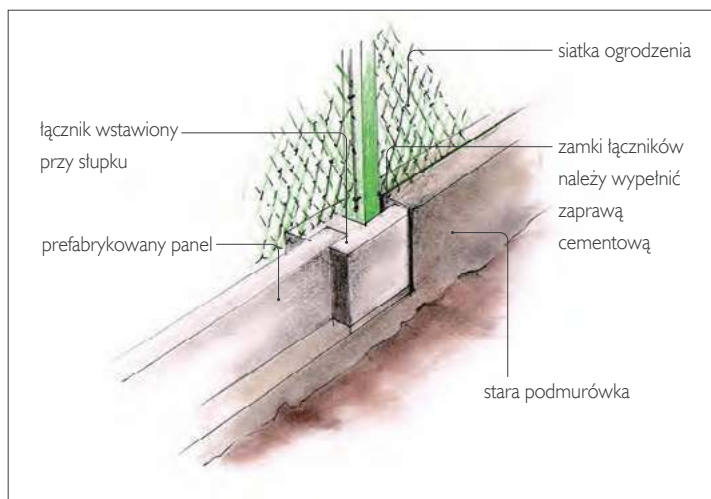
❷ Optymalna metoda remontu to zastąpienie zniszczonej podmurówki elementami prefabrykowanymi.
