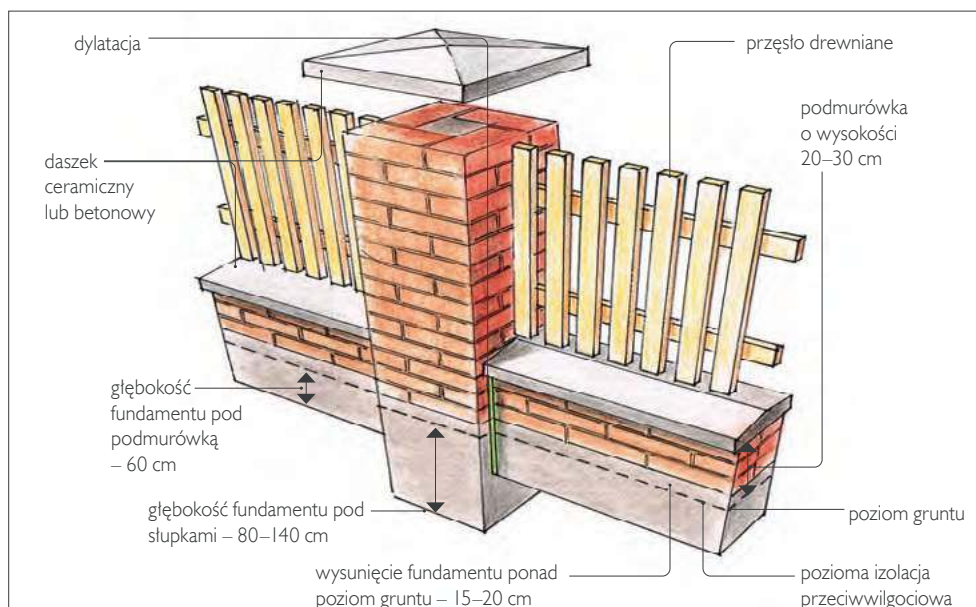
➊ Sposób posadowienia ogrodzenia z murowanym cokołem i słupkami.
