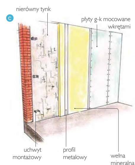
Mocowanie suchego tynku: na klej (a), na pasach z płyt (b), na profilach stalowych (c).
