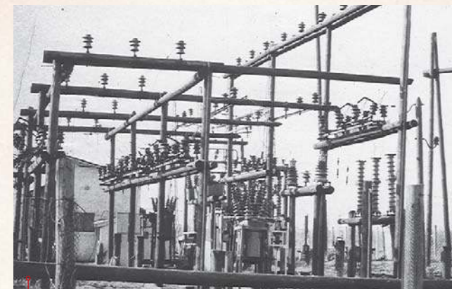
GPZ-1 w pierwszej fazie zabudowy, na drewnianych konstrukcjach
