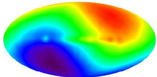
2. Ten obraz kosmicznego tła mikrofalowego pokazuje ruch Ziemi w porównaniu z resztą Wszechświata
