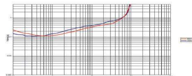
Rys. 3b. THD + N / moc (UL)
