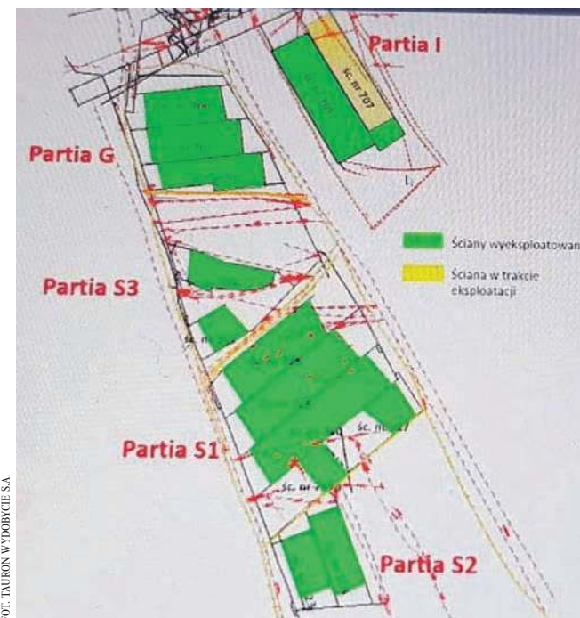
Schemat pokładu 207, w którym trwa eksploatacja
