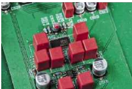
Płytki toru audio są niezależne dla każdego kanału, w roli regulatora głośności zastosowano układ scalony (JRC).
