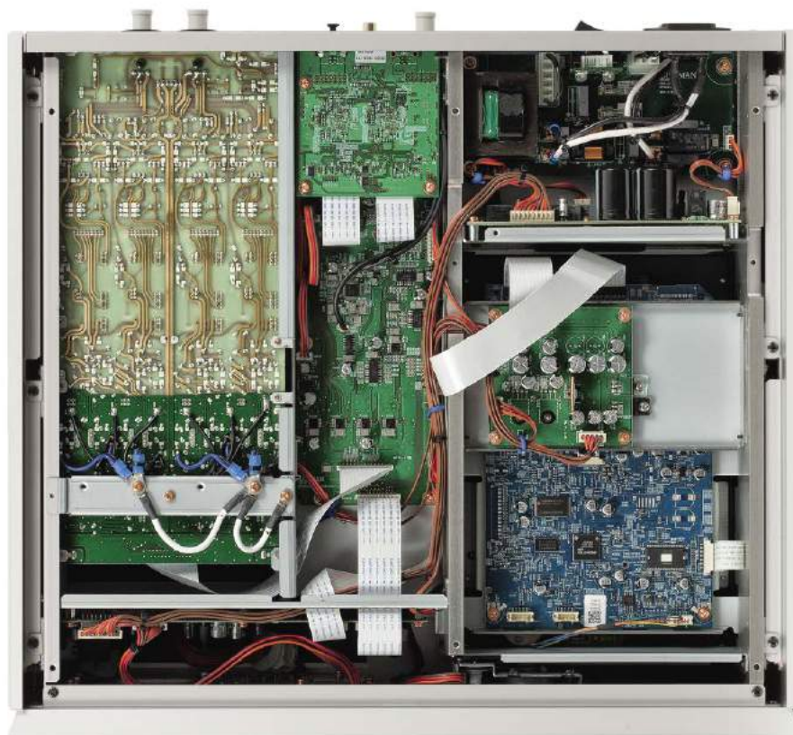
Po odkręceniu dolnej ścianki pojawia się dostęp do elektroniki sterującej i sekcji cyfrowej.
