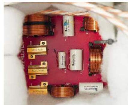
To prawdopodobnie sekcja zwrotnicy dla 18-tek – jak na układ dwóch filtrów dolnoprzepustowych jest bardzo skomplikowana.
