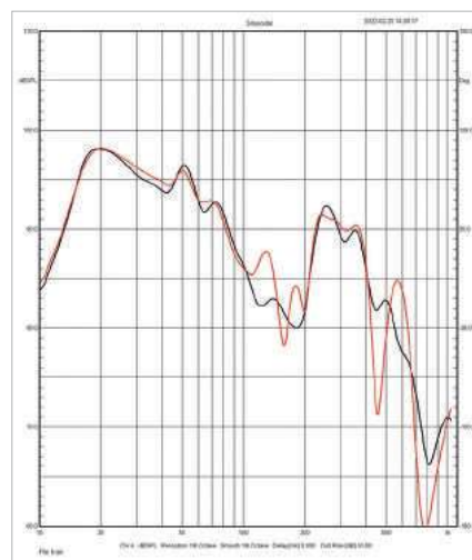
Rys. 6. Charakterystyki ciśnienia z otworu – „z okien” obudowy i bezpośrednio z tuneli.
