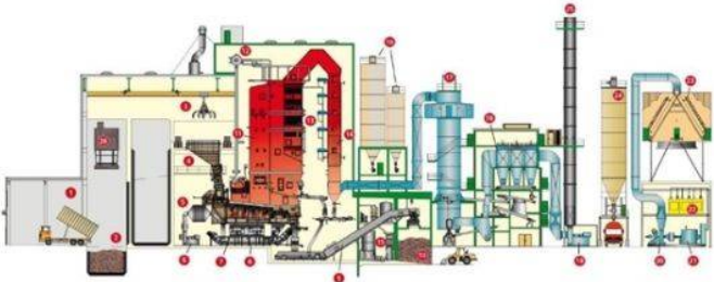
SCHEMAT PRZYKŁADOWEJ INSTALACJI ITPOK
