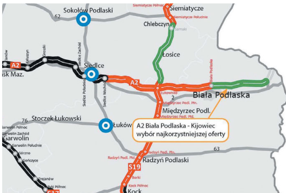
Zgodnie z planem, A2 na omawianym odcinku ma mieć dwie jezdnie z dwoma pasami ruchu oraz rezerwę pod dobudowę trzeciego pasa. Kierowcy mają skorzystać z trasy w 2029 roku
