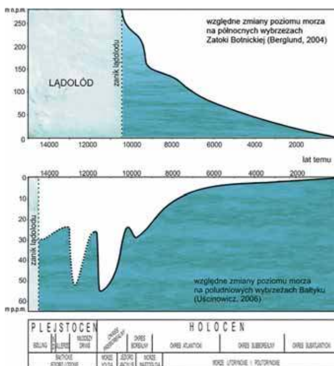
Zmiany poziomu wód Bałtyku od końca plejstocenu do dziś, źródło: PIG-BIP
