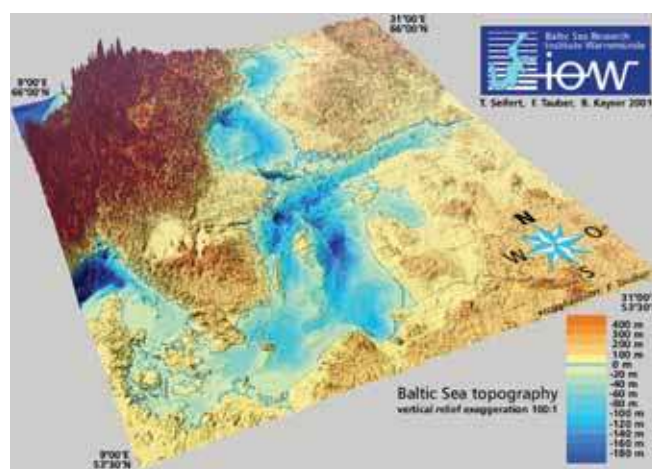
Batymetria Morza Bałtyckiego, źródło: www.io-warnemuende.de
