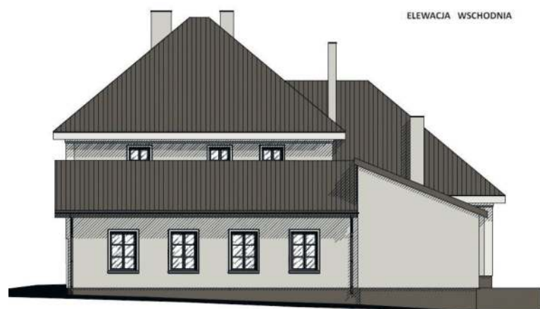
ELEWACJA WSCHODNIA
