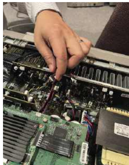
Wnętrze jednego ze wzmacniaczy Marantza; egzemplarz przygotowany do strojenia, w kluczowych miejscach płytek wlutowane są sondy z gniazdami, aby w szybki sposób zmieniać podzespoły, poszukując (na podstawie odsłuchów) najlepszych kombinacji.
