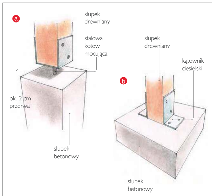
❸ Dwa sposoby osadzenia słupka zadaszenia: przy użyciu kotwy (a), za pomocą kątownika (b).
