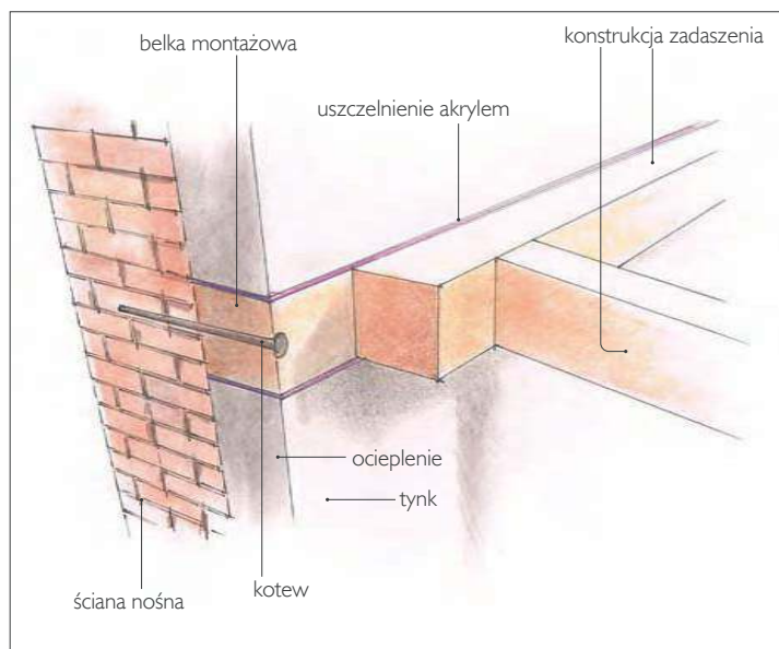
❷ Schemat zamocowania zadaszenia do ściany dwuwarstwowej.
