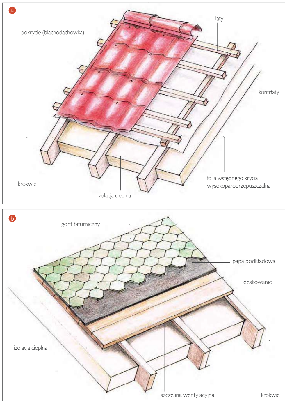
Ruszt z łąt i kontrłąt, czyli rozwiązanie najpopularniejsze (a) i pełne deskowanie – niezbędne pod pokrycie z gontu (b).
