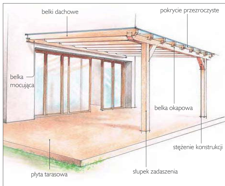
❶ Lekka konstrukcja zadaszenia tarasu.
