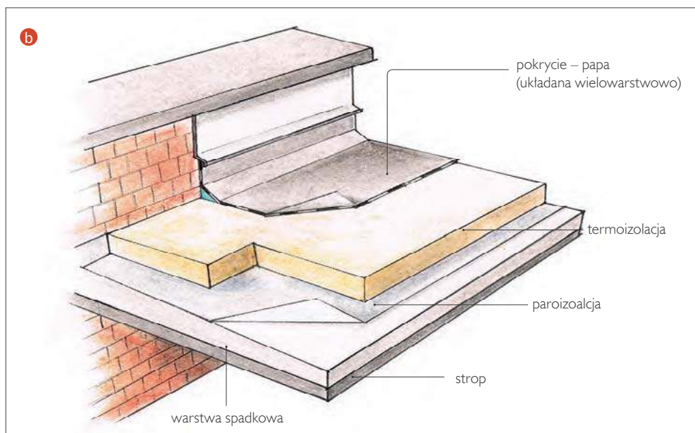
➊ Stropodach wentylowany (a) i niewentylowany (b).
