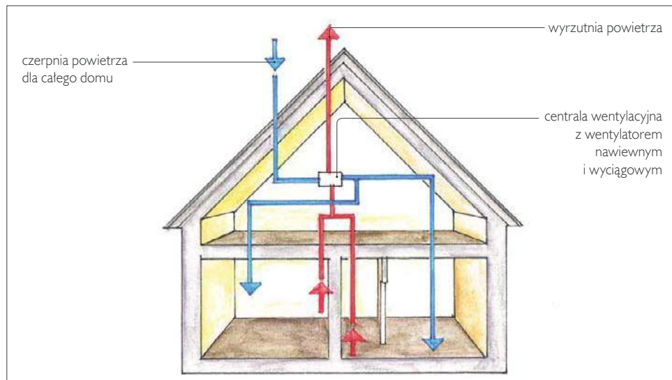
🔗 Sposób działania mechanicznej wentylacji nawiewno-wywiewnej. Tu zarówno za dostarczanie świeżego powietrza, jak i usuwanie zużytego odpowiadają wentylatory.
