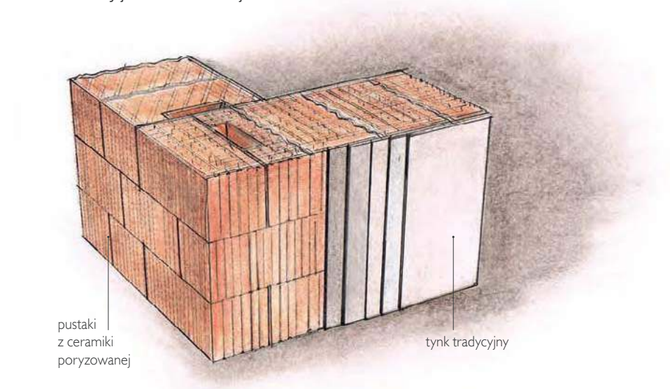
Schemat ściany jednowarstwowej.
