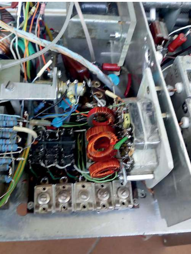
Pokazane są obwody w.cz. dopasowujące z niskiej impedancji wyjściowej KX3 do impedancji w obwodzie siatki sterującej GU-81M
