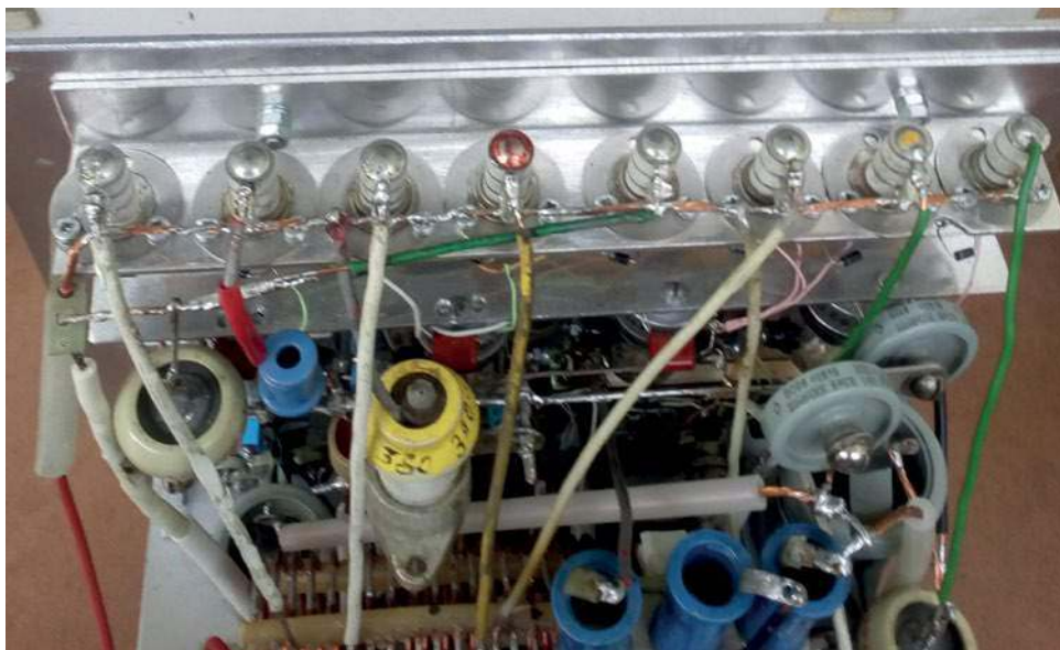
Widok na listwy z zamontowanymi 8 przekaźnikami RF1D-26S (ceramiczne) na wysokie napięcia w.cz. Po zadziałaniu załączają odczepy na cewce L2 oraz kondensatory C antenowe na wyjściu Pi filtra. Poniżej listwa z 4 kondensatorami (szklanymi) próżniowymi B1B-1T1 załączającymi (tym samym sygnałem komutacyjnym) kondensatory C-anodowe Pi filtra. W przypadku najważniejszych dla mnie podpasem DX-owych (3,525 i 3,775 MHz), zarówno kondensatory C-anodowe, jak i C-antenowe składają się z kombinacji ceramicznych kondensatorów o stałych pojemnościach na ten poziom mocy i równolegle do nich dołączane są zmienne kondensatory o regulowanych pojemnościach. Umożliwia to precyzyjne nastrojenie na aktualnie potrzebne wycinki pasma 3,5 CW i 3,8 SSB
