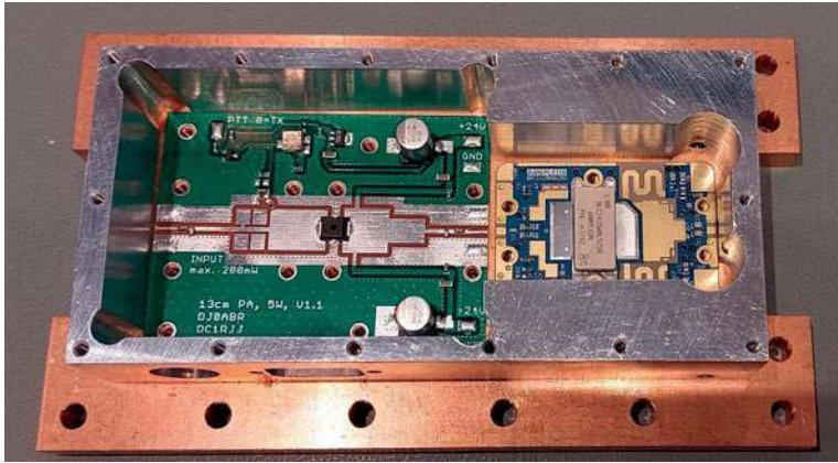
Moduł Ampleon
