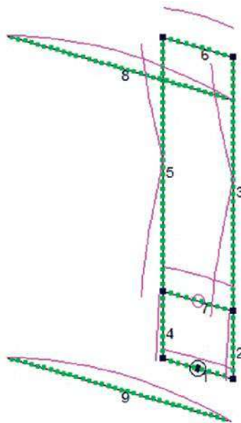
Rys. 3. Elementy konstrukcyjne Hentenny (linie zielone) i rozkłady prądów (linie fioletowe)
