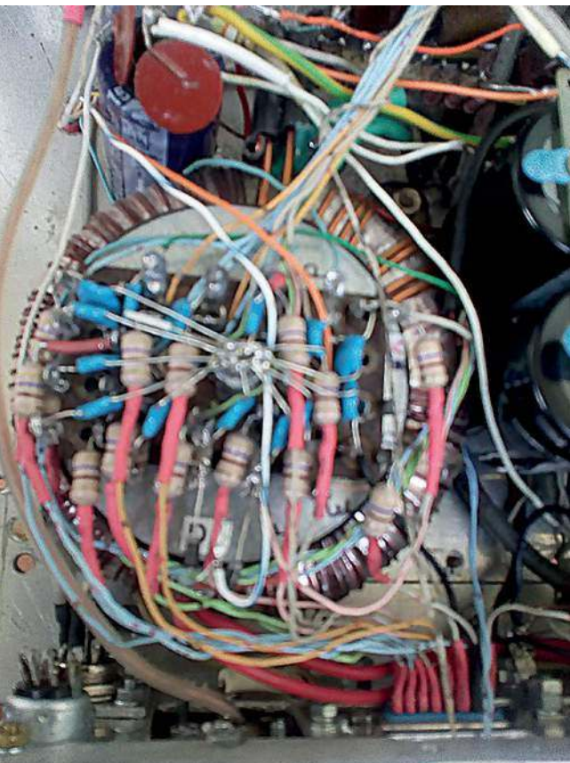
Widoczna jest matryca dolnoprzepustowych filtrów w.c.z. dla (przyszłego) zdalnego sterowania poprzez gniazdo DB15 przez interfejsy zewnętrzne. Pod spodem widoczny fragment transformatora żarzenia katody GU-81M (na toroidzie)
