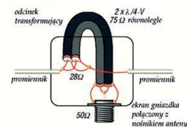
Rys. 2. Sposób dopasowania anteny 28 Ω do linii zasilającej 50 Ω
