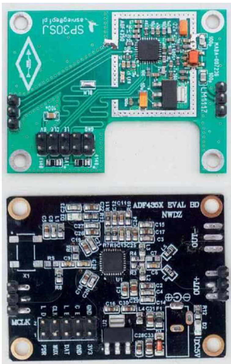
Moduły ADF4350
