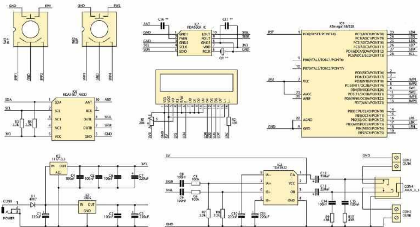
Rys. 3. schemat ideowy radioodbiornika AVT5540
