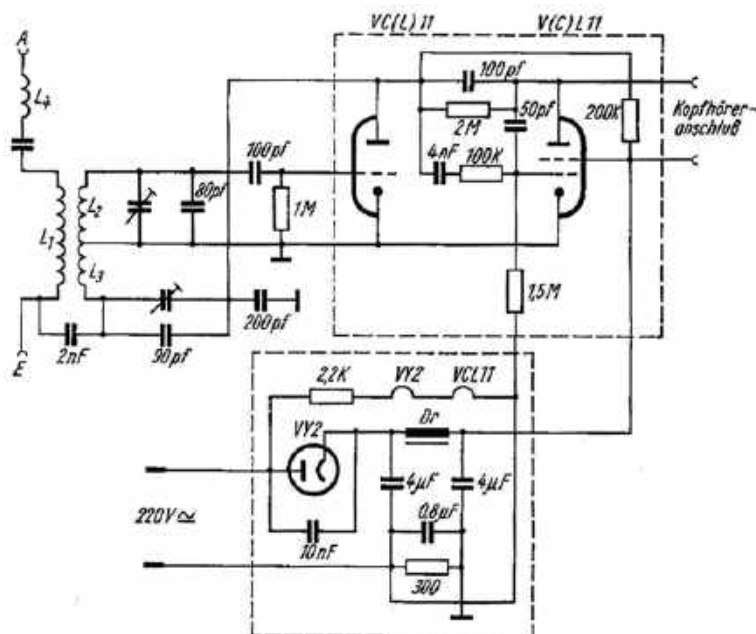
Rys. 2. Odtworzony schemat odbiornika, źródło i.w.
