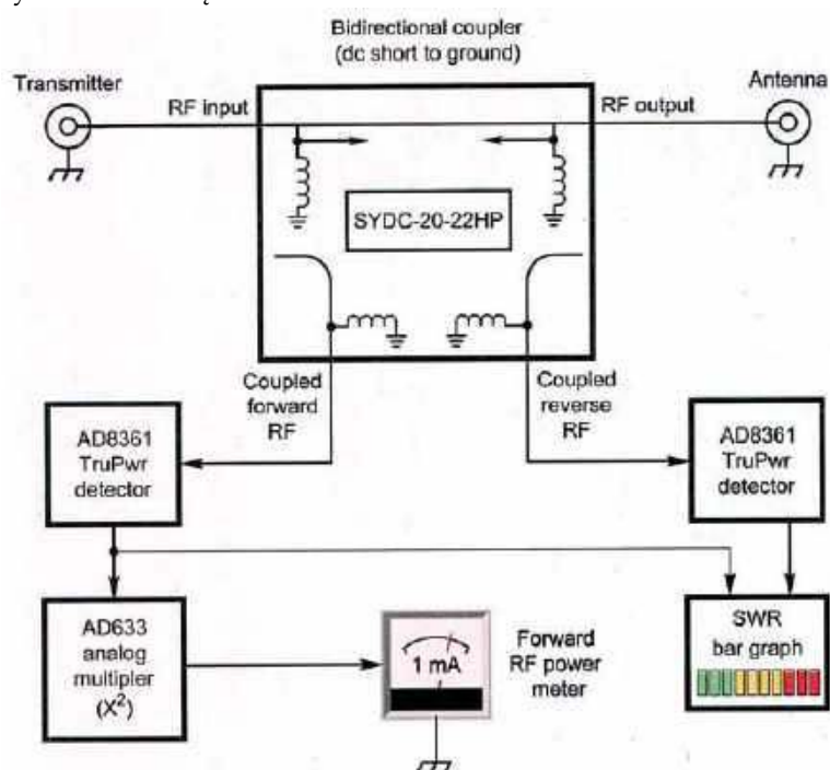
Rys. 5. Schemat blokowy miernika mocy
