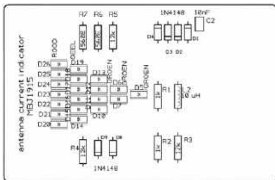
Rys. 4. Szkic rozmieszczenia elementów na PCB
