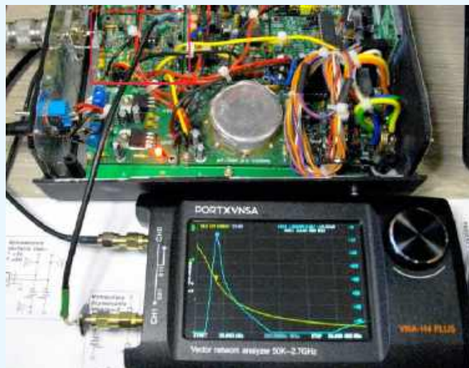
Fotografia 30. Moduł filtrów pasmowych LC w „RX Dosia” podczas pomiarów
