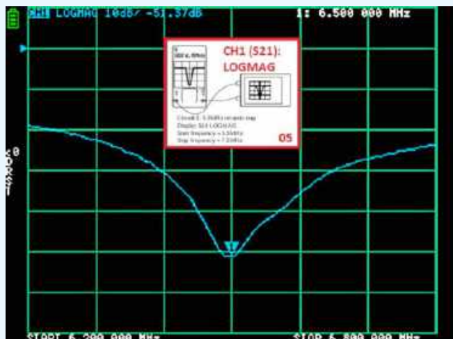
Rysunek 102. Rezultaty pomiarów obwodu nr 5 na płycie RF Demo-Kit
