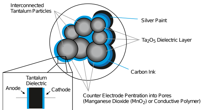
Rysunek 7. Mikrostruktura kondensatora tantalowego [1]
