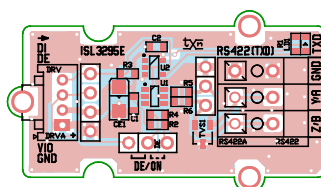
Rysunek 8. Rozmieszczenie elementów modułu Grove_RS422T_ISL3295E
