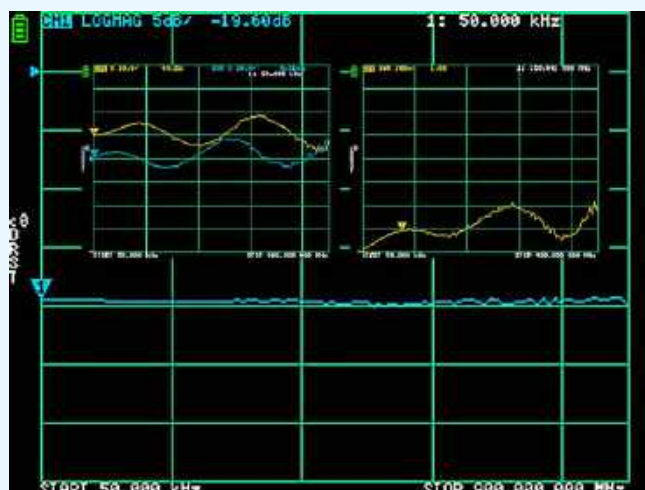
Rysunek 127. Charakterystyki częstotliwościowe: tłumienności, SWR oraz R i X tłumika stałego przy A=20 dB
