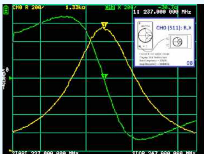
Rysunek 104. Rezultaty pomiarów obwodu nr 8 na płycie RF Demo-Kit
