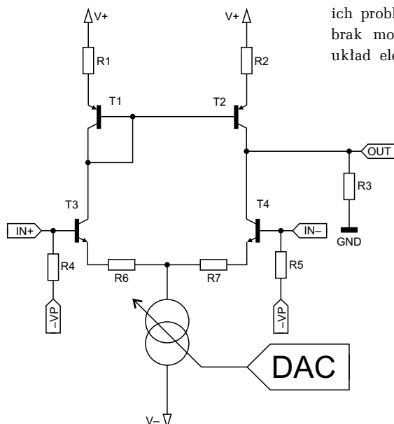
Rysunek 1. Uproszczony schemat regulatora wzmacnienia z układem różnicowym
