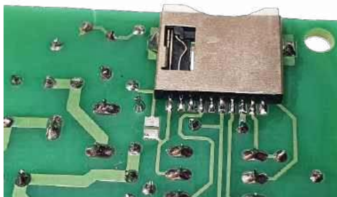
Fotografia 1. Widok przylutowanego złącza karty microSD
