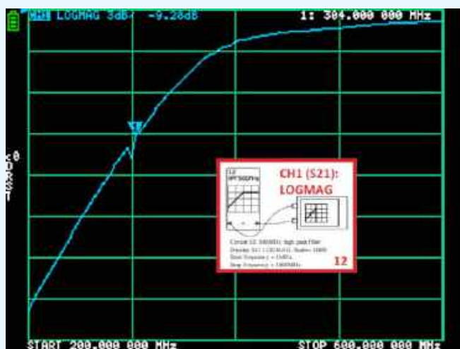
Rysunek 106. Rezultaty pomiarów obwodu nr 12 na płycie RF Demo-Kit
