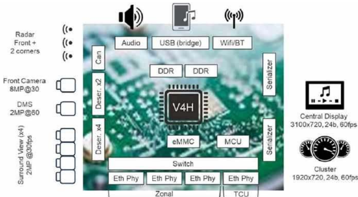
Rysunek 10. Zasoby sprzętowe układu V4H od Renesas ( https://www.renesas.com/en/blogs/exploring-entry-fusion-application-architecture-and-cost-effective-solution-utilizing-r-car-v4h?srltid=AfmBOop_zsvMCSVPgKWPVYES5Kr9hcnT-SB8FkSCd7qQsDiuqgN5Vq4a )
