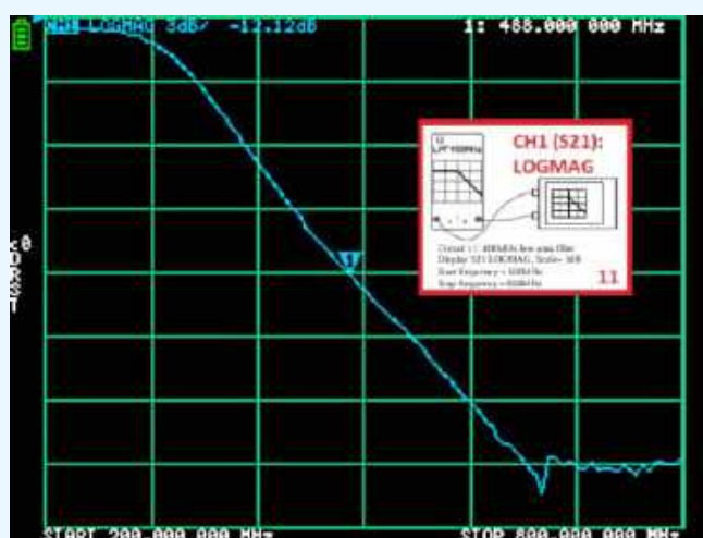
Rysunek 105. Rezultaty pomiarów obwodu nr 11 na płycie RF Demo-Kit
