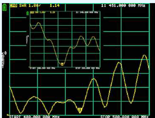
Rysunek 111. Wykresy parametrów SWR dla pasm VHF/UHF anteny NAGOYA NL-770R
