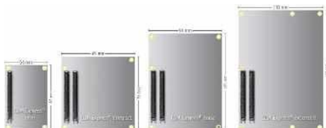
Rysunek 15. Budowa modułów SoM w standardzie COM Express wraz z rozmieszczeniem złączy ( https://en.wikipedia.org/wiki/COM_Express#/media/File:COM_Express_form_factor_comparison.jpg )
