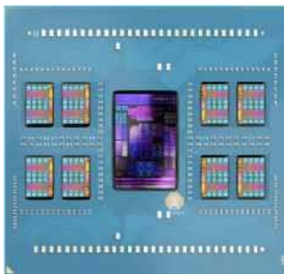
Fotografia 2. Procesor AMD EPYC Bergamo, wykonany z użyciem chipletów, który ma aż 128 rdzeni ( https://wccftech.com/amd-epyc-bergammo-cpu-die-detailed-16zen-4c-vindhya-cores-per-ccd-35-percent-smaller-core-area/ )
