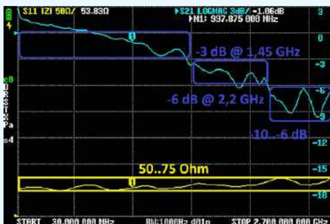
Rysunek 132. Charakterystyki częstotliwościowe tłumienia i SWR wzmacniacza LNA 30...4000 MHz/40 dB
