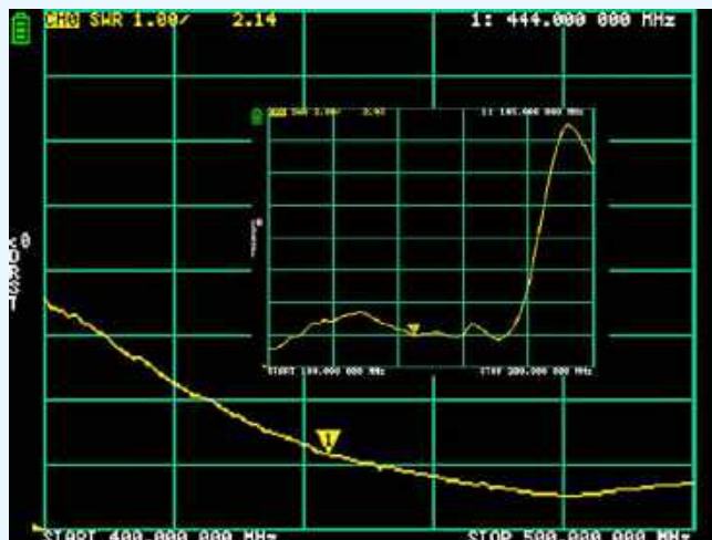
Rysunek 110. Wykresy parametrów SWR dla pasm VHF/UHF anteny DIAMOND RH901S
