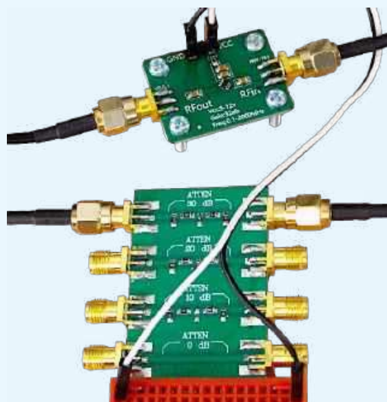
Fotografia 36. Wzmacniacz LNA 0,1...2000 MHz/30 dB
