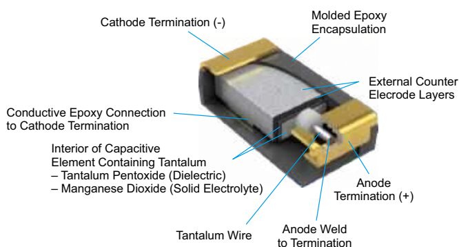
Rysunek 3. Budowa kondensatora tantalowego w obudowie SMD [1]
