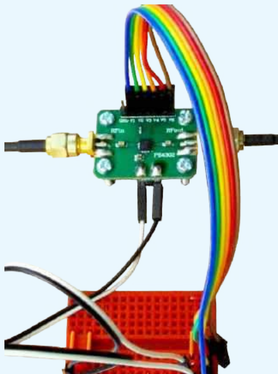
Fotografia 34. Tłumik regulowany z układem scalonym PE4302
