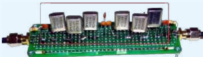
Fotografia 29. Prototyp jednego z badanych filtrów SSB
