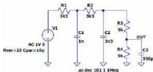
Rysunek 2. Schemat symulacyjny dolnoprzepustowego filtra RC
