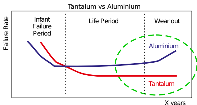
Rysunek 4. Odsetek uszkodzeń w funkcji czasu [1]
