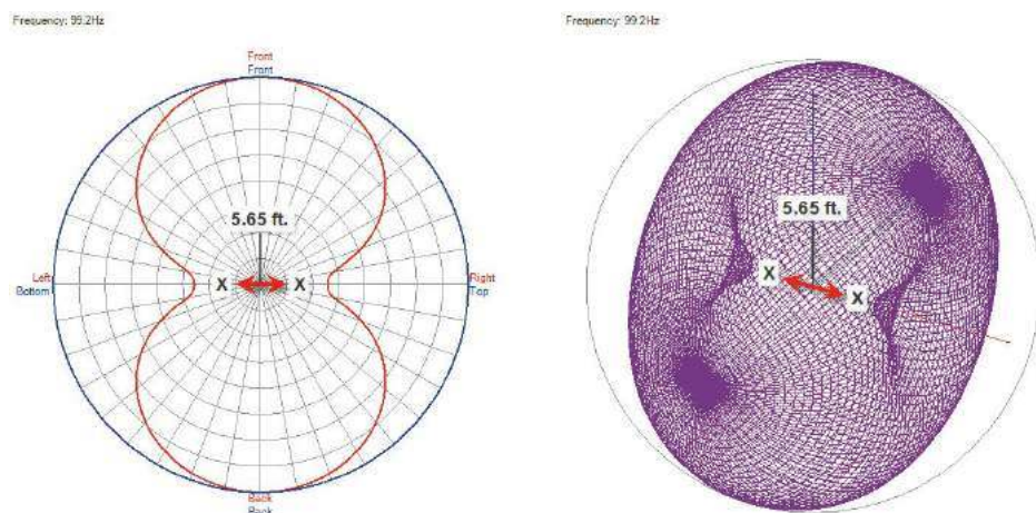
Rysunek 11. Dwa idealne punktowe, wszechkierunkowe źródła umieszczone w odległości 172 cm (5 ms różnicy czasowej przy prędkości dźwięku 344 m/s).
