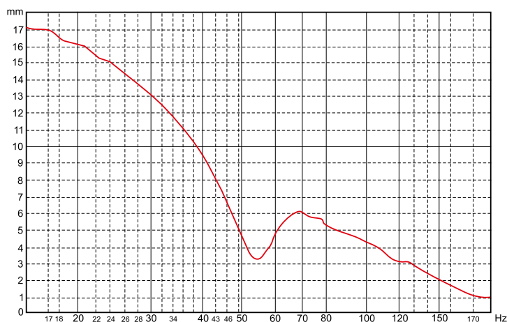
Rysunek 6. Przeskalowany wykres wychylenia membrany 15-calowego woofera w obudowie bass-reflex, zasilanego przemiennym sygnałem sinusoidalnym o napięciu 63,2 V RMS .
