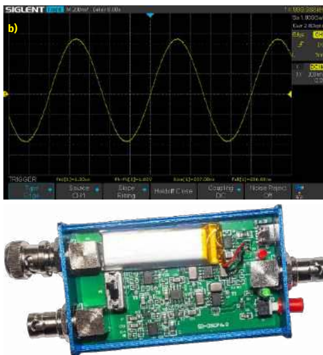
Fotografia 2. Wnętrze sondy, wyjątkowo skomplikowane, biorąc pod uwagę, że za realizację funkcji wzmacniacza różnicowego odpowiada w istocie jeden układ scalony (INA849)
