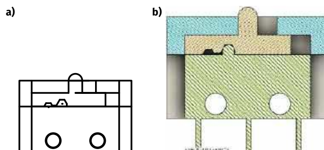
Rysunek 2. Podstawowy przełącznik suwakowy: szkic (a) i przekrój modelu (b)
