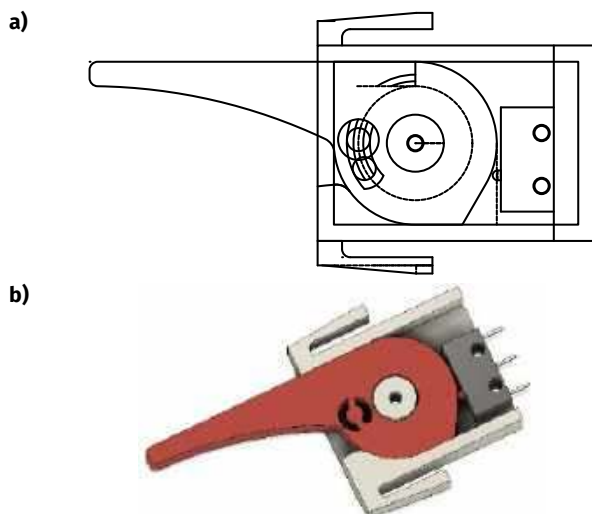
Rysunek 5. Przetłaczni dźwigniowy: szkic (a) i dwa główne elementy przetłaczni wraz z modelem mikroprzetłaczni (b)
