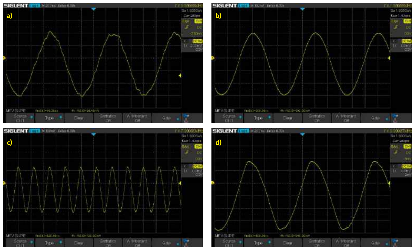
Rysunek 3. Pomiar sondy w trybie single-ended przy wzmacnieniu 100×: sygnał źródłowy o częstotliwości 10 MHz i amplitudzie 10,4 mVp-p (a), sygnał wyjściowy przy 2 MHz (b), 8 MHz (c) i 10 MHz (d)
