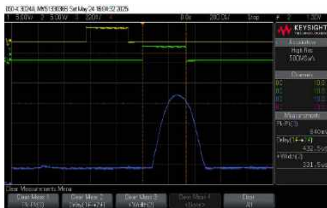
Rysunek 6. Odpowiedź czujnika w czystym powietrzu
