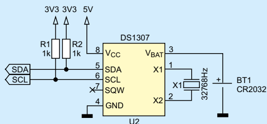
Rysunek 1. Przykładowy schemat implementacji układu DS1307
