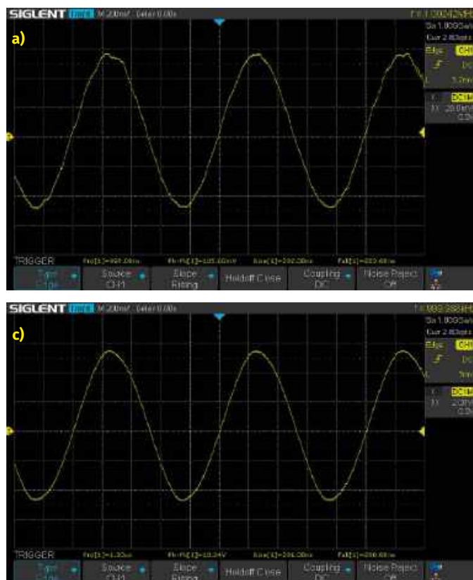
Rysunek 6. Ten sam test, ale tym razem sygnały są w przeciwfazie, wzmocnienie 1\times (a), 10\times (b) oraz 100\times (c). Sonda pracuje poprawnie, a zakłócenia, które – wydawałoby się – powinny zdominować sygnał, niemal kompletnie zniknęły
