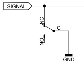
Rysunek 2. Zwieranie sygnału przekaźnikiem do masy – funkcja „mute”
