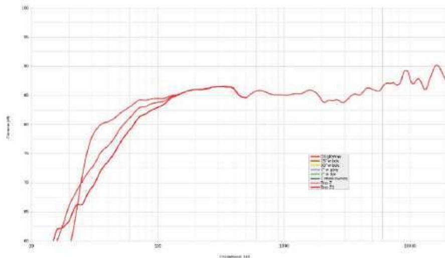
Rysunek 18. Monitor Audio Gold 300 G6, charakterystyka w pełnym paśmie, uzyskana łąčeniem pomiarów w polu bliskim i MLS, przy 500 Hz, dla trzech wariantów strojenia obudowy
