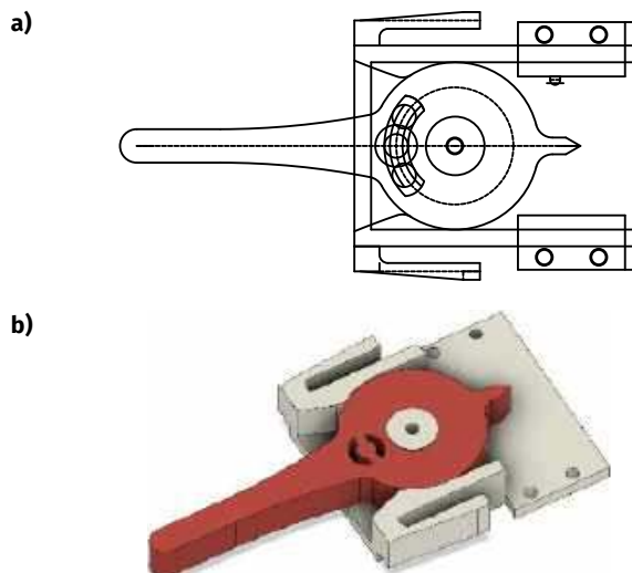
Rysunek 7. Przetłaczni dźwigniowy w trzech pozycjach: szkic (a) i dwa główne elementy przetłaczni (b)
