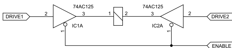
Rysunek 5. Proste sterowanie przełącznika bistabilnego
