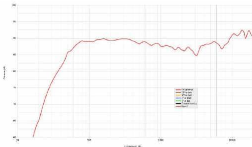
Rysunek 12. Paradigm Founder 100F, charakterystyka w pełnym paśmie, uzyskana łąčeniami pomiarów w polu bliskim i MLS, przy 500 Hz
