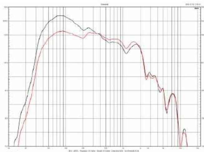
Rysunek 4. Sonoro Grand Orchestra, charakterystyka wypadkowa źródeł niskich częstotliwości, przed (czarna) i po korekcie baffle-step (czerwona)
