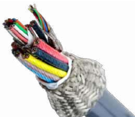
Fotografia 9. Przewód o wielopoziomowej strukturze grupowej marki NEWT
