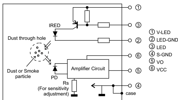
Rysunek 2. Schemat wewnętrzny czujnika GP2Y1010AU0F [2]
