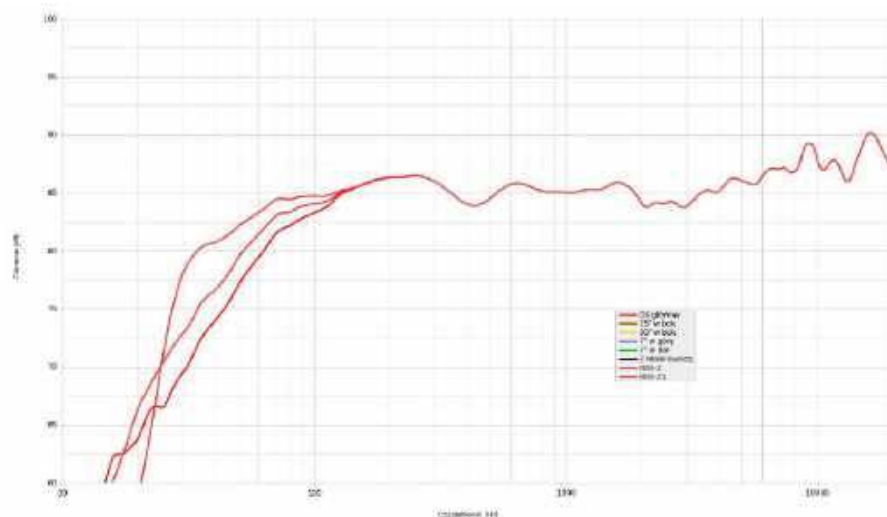
Rysunek 17. Monitor Audio Gold 300 G6, charakterystyka w pełnym paśmie, uzyskana łąčeniem pomiarów w polu bliskim i MLS, przy 250 Hz, dla trzech wariantów strojenia obudowy
