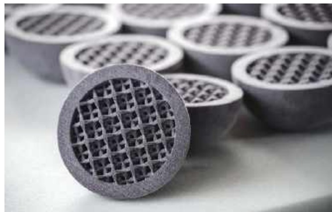
Fotografia 6. Detale wytworzone metodą natryskiwania spoiwa i spiekania ( https://t.ly/jenJ4 )
