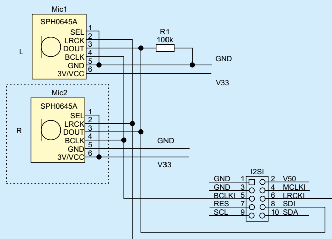
Rysunek 8. Schemat podłączenia mikrofonów MEMS do złącza I 2 S
