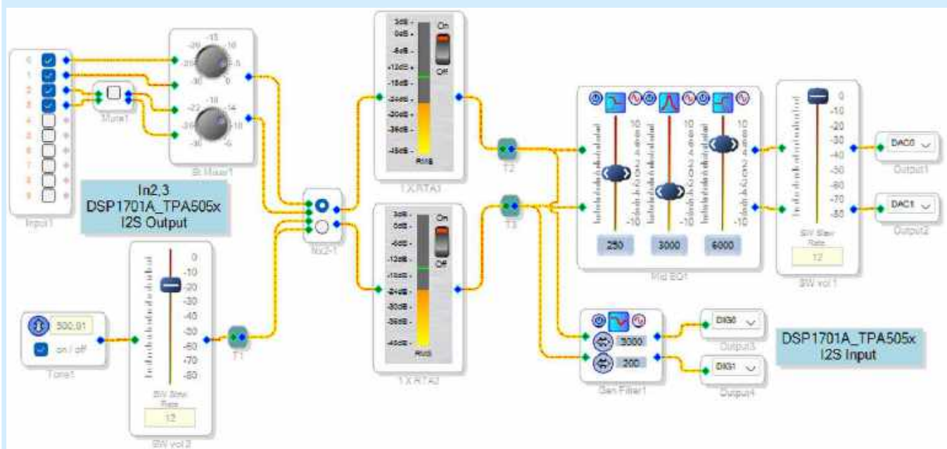
Rysunek 14. Schemat aplikacji przykładowej ADAU1701_MK2_Cz5_ProjektTestowyI2SDelay.dspproj
