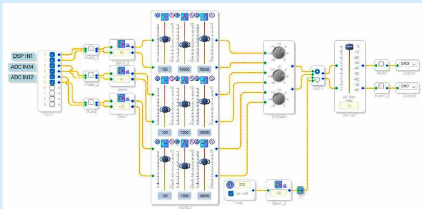
Rysunek 16. Schemat aplikacji przykładowej ADAU1701_MK2_Cz5_ProjektTestowyTDMADC.dspproj
