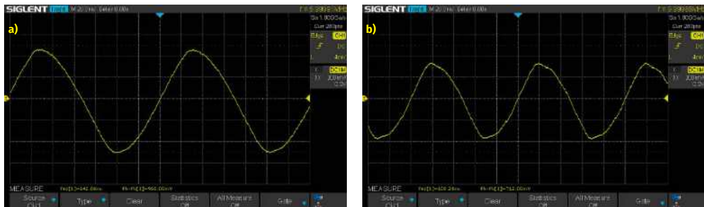
Rysunek 2. Pomiar sondy w trybie single-ended przy wzmacnieniu 10× z użyciem sygnału z rysunku 1a: sygnał wyjściowy przy 9 MHz (a) i 10 MHz (b)
