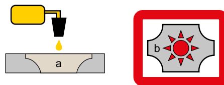
Rysunek 6. Etapy wytwarzania metodą natryskiwania spoiwa i spiekania: wytworzenie kształtki (a), spiekanie kształtki (b)
