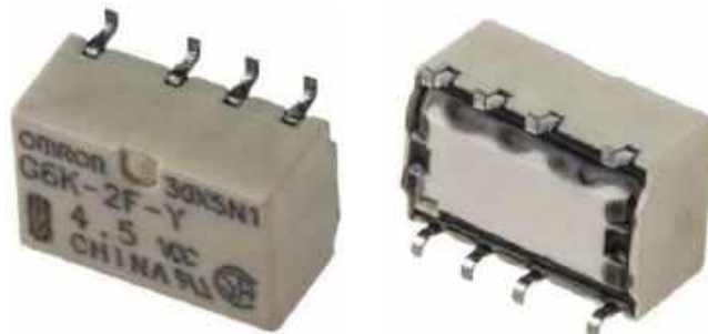
Fotografia 1. Przekaźnik sygnałowy bez wymaganej minimalnej mocy przełączanej [2]
