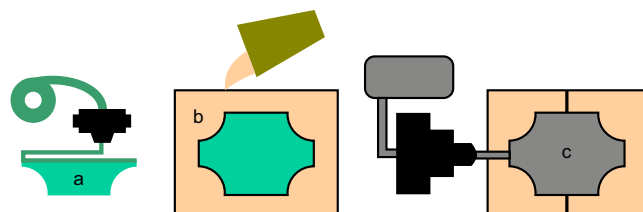
Rysunek 1. Etapy wytwarzania metodą odlewania z wosku traconego: druk modelu (a), odlewanie formy (b), odlewanie elementu (c)
