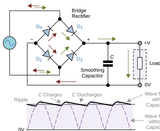
Rysunek 1. Schemat prostownika dwupołówkowego z filtrem oraz przykładowy przebieg napięcia wyjściowego
