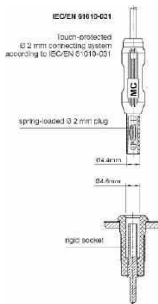
Rysunek 4. Wymiary złączy bezpiecznych w rozmiarze 2 mm ( https://t.ly/DAJD1 )
