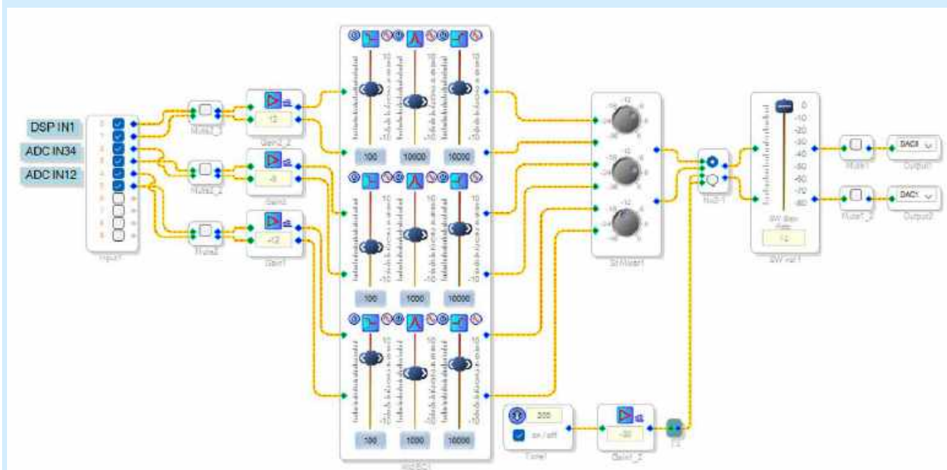
Rysunek 16. Schemat aplikacji przykładowej ADAU1701_MK2_Cz5_ProjektTestowyTDMADC.dspproj
