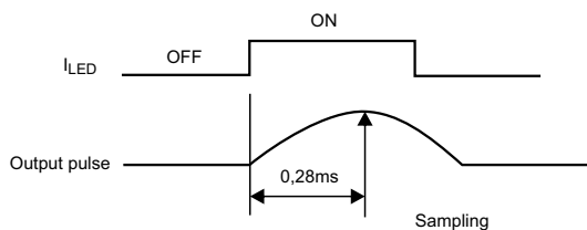
Rysunek 3. Sposób pomiaru sygnału z czujnika [2]
