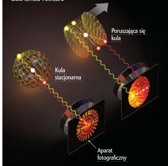
Efekt Terrella-Penrose'a
