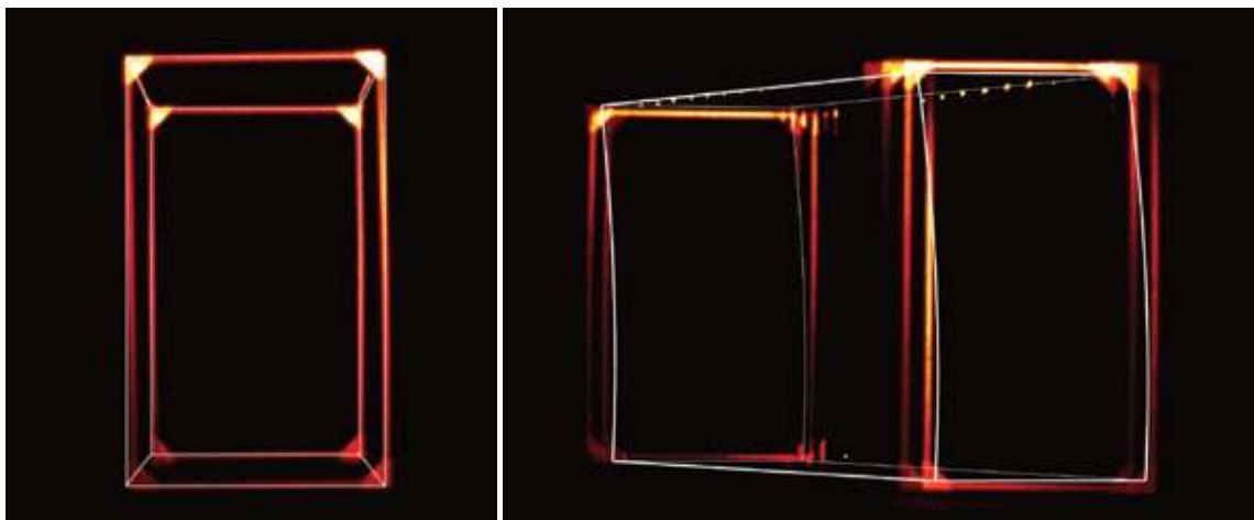
Na fotografiach z eksperymentu widać efekt obrotu Terrella-Penrose'a sześcianu skróconego przez efekt Lorentza (z lewej), który dzięki sprytnym sztuczkom wydawał się poruszać z prędkością równą 80% prędkości światła.
