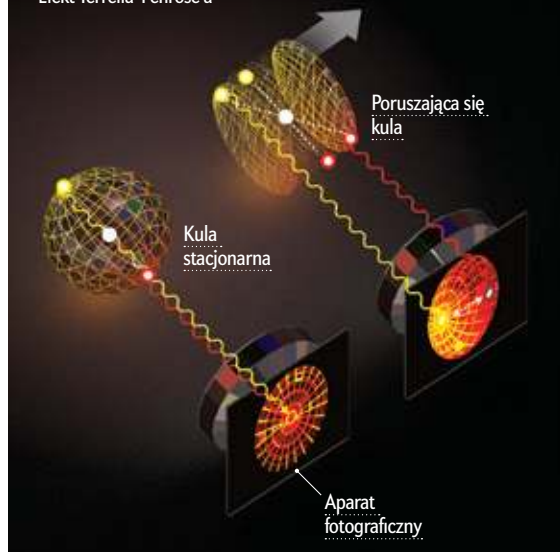
Efekt Terrella-Penrose'a
