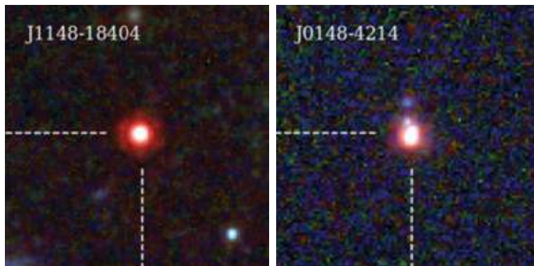
Od momentu uruchomienia Kosmiczny Teleskop Jamesa Webba odkrył w przestrzeni kosmicznej dziesiątki tajemniczych czerwonych plamek. Małe Czerwone Kropki zaczęły pojawiać się około 600 mln lat po Wielkim Wybuchu i wydaje się, że zniknęły około 1,5 mld lat po nim.
