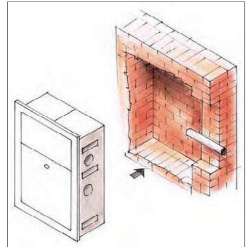
➋ Montaż podtynkowy.
