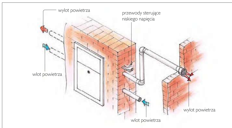
Wydech powietrza na zewnątrz budynku.
