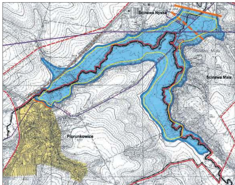
Zbiornik ma się znajdować na granicy gmin Prudnik i Korfantów
