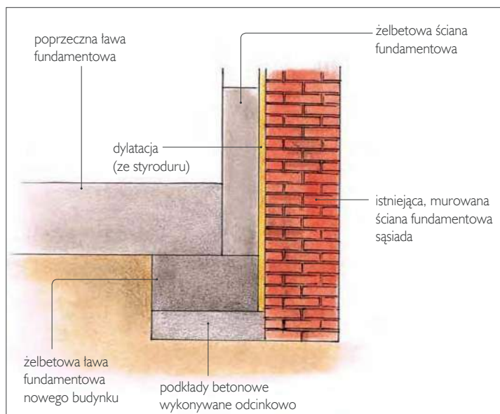
📍 Fundamentowanie przy dobudowie bliźniaczej do istniejącego budynku – jedna połówka bez podpiwniczenia, druga z mieszkaniem w suterenie.
