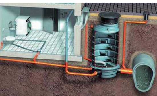
Zawór zwrotny można też zamontować w studzience przyłączeniowej przed budynkiem. KESSEL
