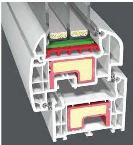
❶ Energooszczędne okna z PVC mogą mieć komory wypełnione pianką poliuretanową. MS WIĘCEJ NIŻ OKNA
