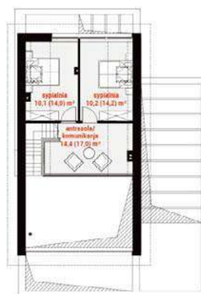
RZUT PODDASZA
