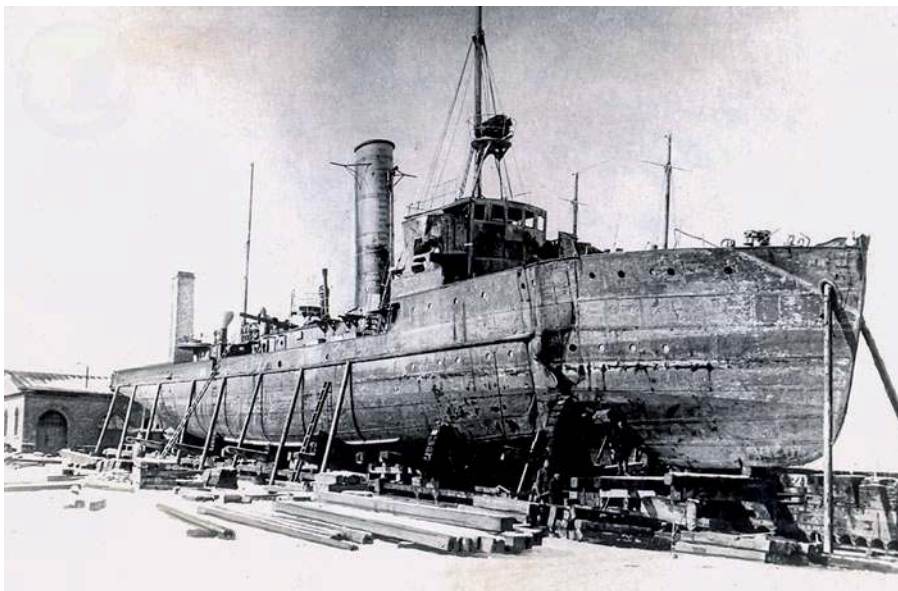
▲ Niemiecki trałowiec M 68, który 29 października 1917 roku wszedł na minę w rejonie Dyneburga i zatonął. 15 marca 1919 roku został podniesiony z dna i odholowany do Rygi. Pomimo, że jednostka nie nadawała się do działań została wpisana na stan jako Sarkanā Latvija (Czerwona Łotwa).
