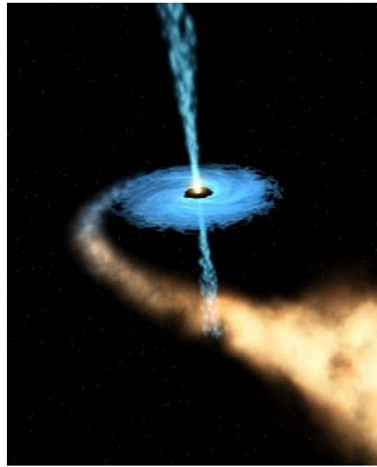
Rys. 1. Dysk akrecyjny, źródło ilustracji: https://pl.wikipedia.org/wiki/Dysk_akrecyjny
