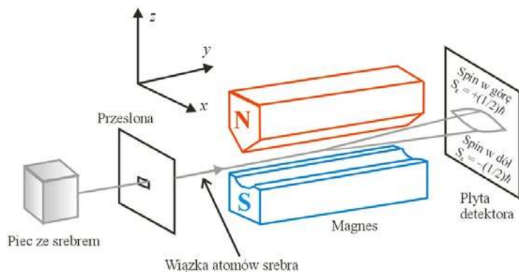
Rysunek 1. Schemat doświadczenia Stern-Gerlach.
