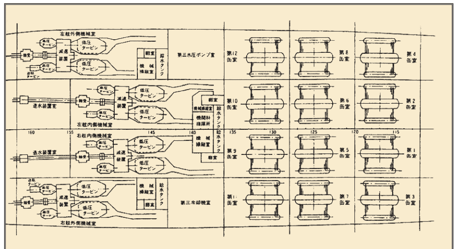
Napęd pancernika Musashi – kotłownie z kotłami parowymi 12-Shiki Ro Gō Kampon – Kansei Honbu Dai i maszynownie z turbozespołami parowymi Nagasaki Kampon 2 Gata T1.
