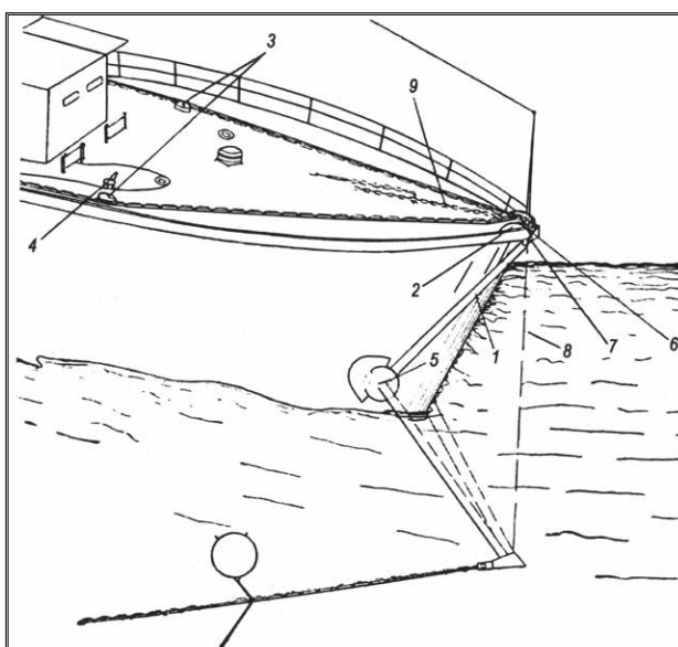
Rysunek przedstawiający zasadę montowania na dziobie ochraniaczy przeciwmicznych.
