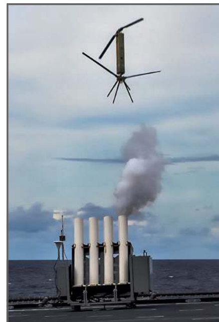
Próby elementów aktywnego systemu w postaci wyrzutni celów pozornych na pokładzie LCS-2. Docelowo jednostki miały dysponować wyrzutniami Mk 53 do pocisków Nulka produkcji BAE Systems Australia, jednak dotąd niewiele z okrętów serii LCS je otrzymało (o ile w ogóle).
