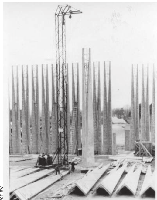
Ustawianie gotowych prefabrykatów odbywało się przy pomocy... ręcznego żurawia, poruszanego przez minimum sześciu mężczyzn. Wszystkie prefabrykaty boczne, sufitowe oraz słupy nośne wykonywano na miejscu budowy
