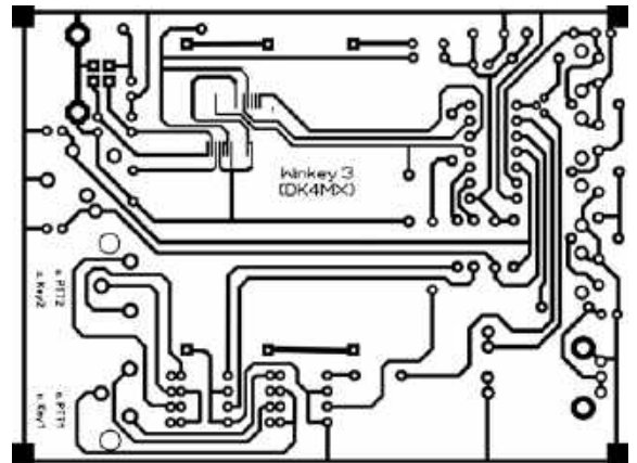
Rys. 5. Płytkę drukowaną Winkey-Keyer 3
