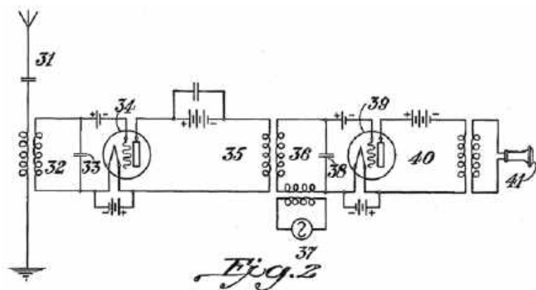
Rys. 2. Schemat mieszacza-demodulatora ze wzmacniaczem w.cz.
