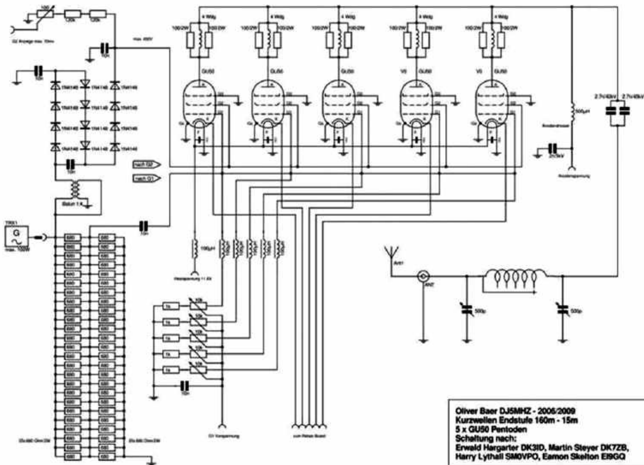
Rys. 3. Schemat ideowy wzmacniacza G2DAF na 5×GU50
