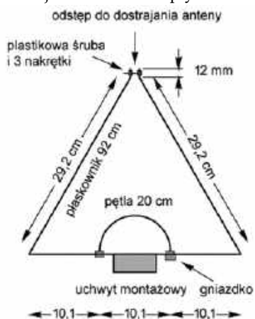
Rys. 1. Wymiary anteny
