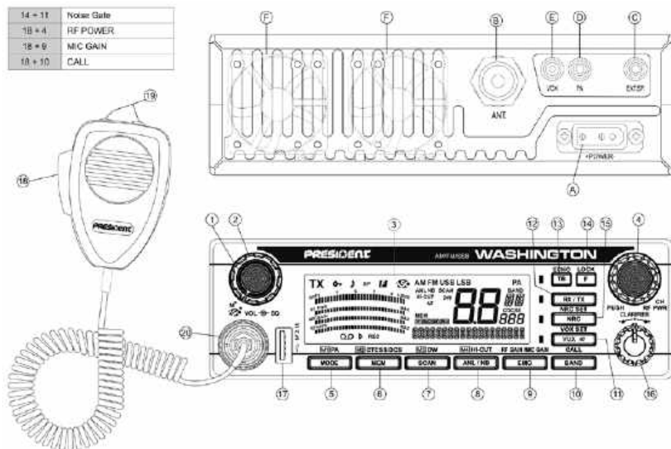
Rys. 1. Elementy regulacyjne i gniazda podłączeniowe
