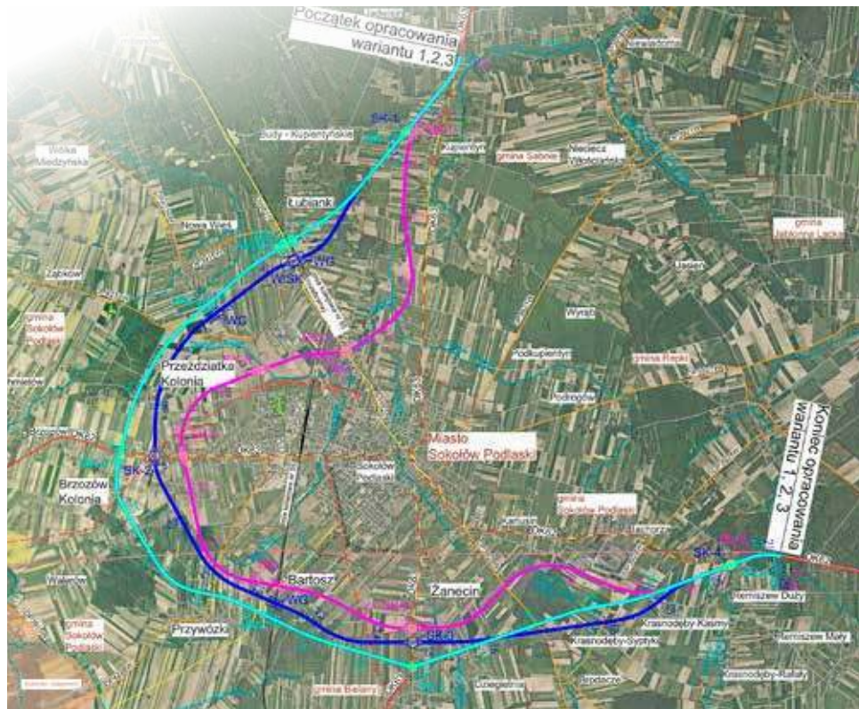
Plan uwzględniający przebieg 3 zaproponowanych wersji obwodnicy
