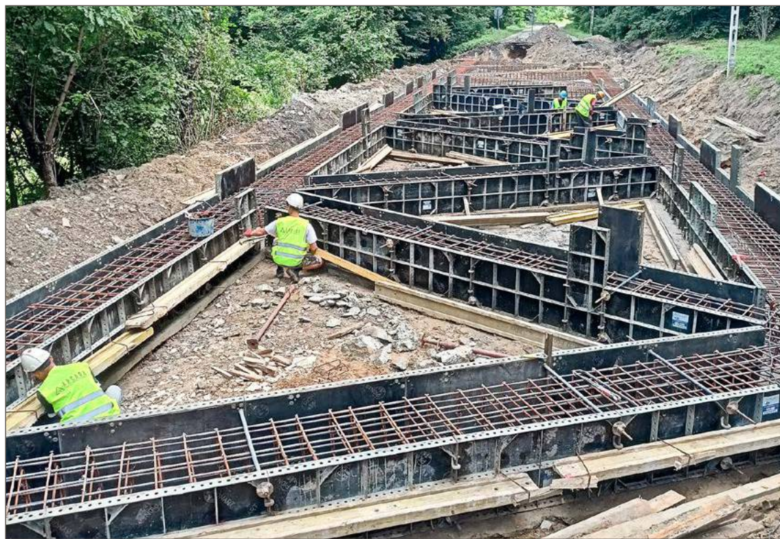
W Połomii, gdzie trwa budowa konstrukcji oporowej, drogę trzeba było zupełnie zamknąć dla ruchu.
