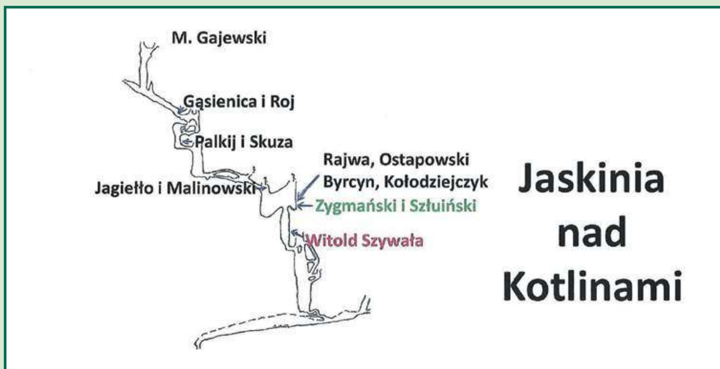
Przekrój jaskini z rozmieszczeniem na wyprawie ratowników - kolor czarny i grotołazów - zielony i czerwony.
