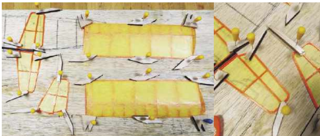
Mocowanie skrzydeł i stateczników po zaimpregnowaniu
