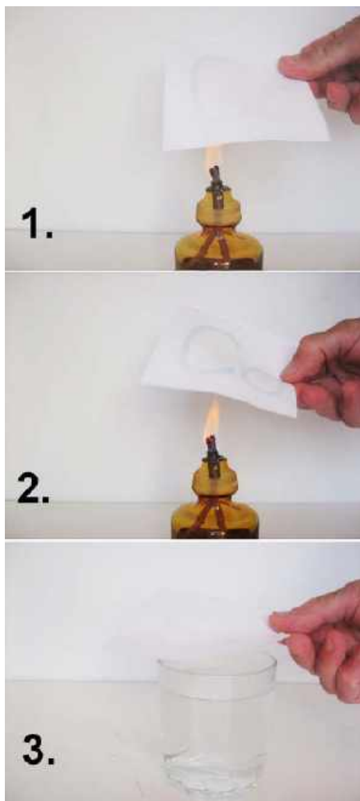
1. Napis sporządzony roztworem chlorku kobaltu(II) po umieszczeniu nad płomieniem palnika (1) ujawnia się w postaci niebieskich liter (2). Działanie pary wodnej ponownie ukrywa napis (3)
