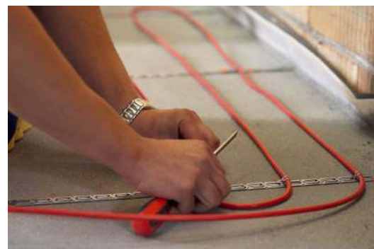
Układanie przewodów grzejących. DANFOSS/DEVI
