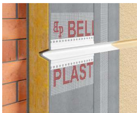
📍 Listwa z PVC do boniowania trójkątna – rąbek wklęsły. BELLA PLAST
