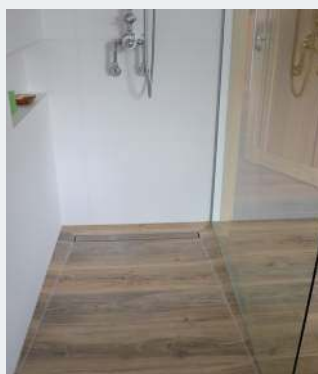
🔗 Wokół odpływu liniowego wyprofilowano kopertowy spadek.
