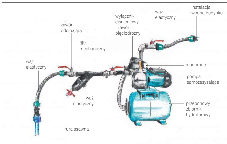
Schemat budowy układu z hydroforem przeponowym.
