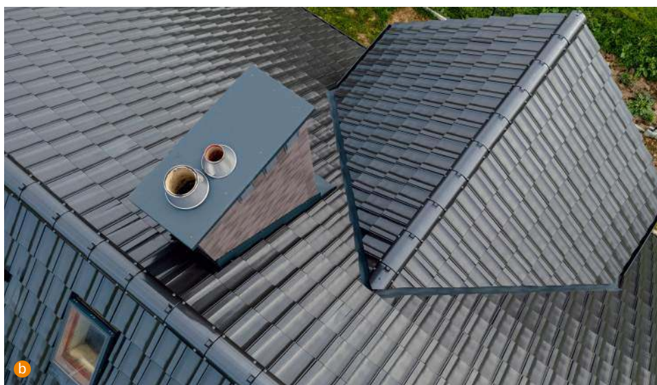
📍 Dach pokryty dachówką cementową (a) i ceramiczną (b). CREATON POLSKA
