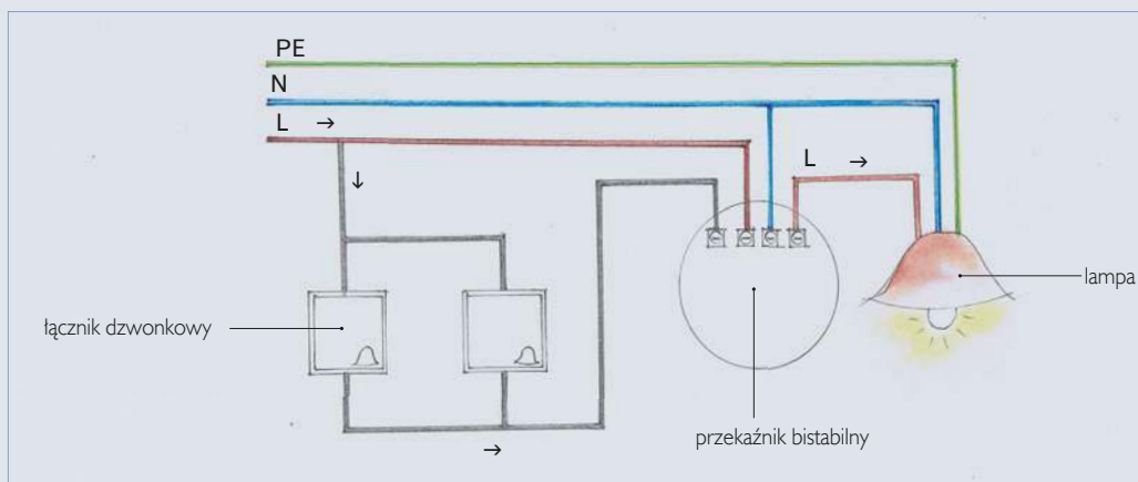
🔧 Układ połączeń w obwodzie z przełącznikiem bistabilnym i łącznikami dzwonkowymi. L – żyła fazowa; N – żyła neutralna; PE – żyła ochronna.
