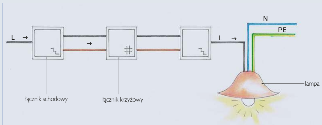
🔧 Układ połączeń w obwodzie z łącznikami schodowymi i krzyżowymi. L – żyła fazowa; N – żyła neutralna; PE – żyła ochronna.
