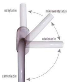
🔗 Różne pozycje klamki, w zależności od pożądanego efektu otwarcia skrzydła. OKNOPLAST, REM II
