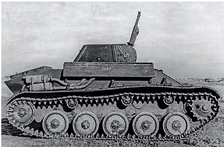
▲ Czołg przeciwlotniczy T-70-Z w profilowym ujęciu z karabinami maszynowymi maksymalnie podniesionymi. Tu dobrze widać, że wykorzystano znaczną część oryginalnej wieży czołgowej. Na wlocie powietrza do silników (zespół napędowy z T-70) widać numer seryjny, ale chyba niepełny, czołgu użyczającego swój kadłub. Pod wlotem widoczne są tłumiki.
