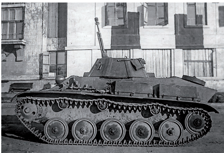
▲ Stojący na dziedzińcu zakładów GAZ czołg przeciwlotniczy T-90. Widok na lewą burtę. Dla zdjęcia lufy ustawiono do maksymalnego kąta podniesienia. Zdjęcie przypuszczalnie pochodzi z okresu prób zakładowych. Z boku kadłuba, pod przednią częścią wieży, widać numer czołgu wykorzystanego do budowy prototypu – 7207789, gdzie 7 oznacza typ, 2 oznacza 1942 rok, 07 oznacza lipiec a 789 to numer podwozia.
