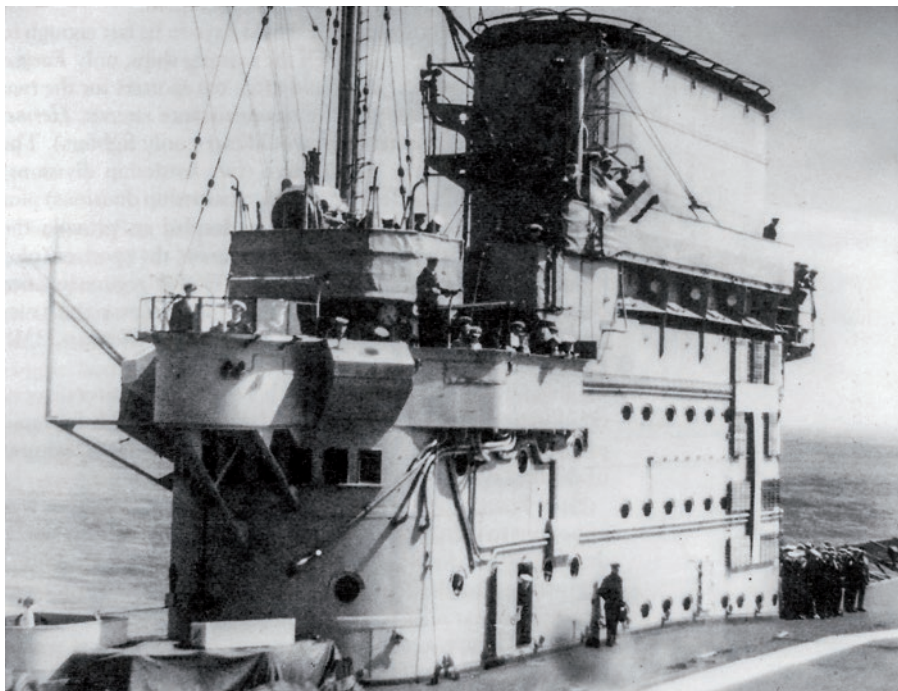
▲ Niewielka „wysepka” typu „kominowego” lotniskowca Courageous .
