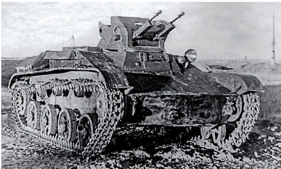
▲ Czołg przeciwlotniczy T-60-Z. Na tym zdjęciu dobrze widać pancerną osłonę uzbrojenia i zakres wykorzystania elementów oryginalnej wieży czołgowej. Miało to zmniejszać koszt adaptacji czołgu, który w tym czasie utracił wartość bojową. Dolna przednia płyta kadłuba została wzmocniona dodatkowym pancerzem o grubości 15 mm.
