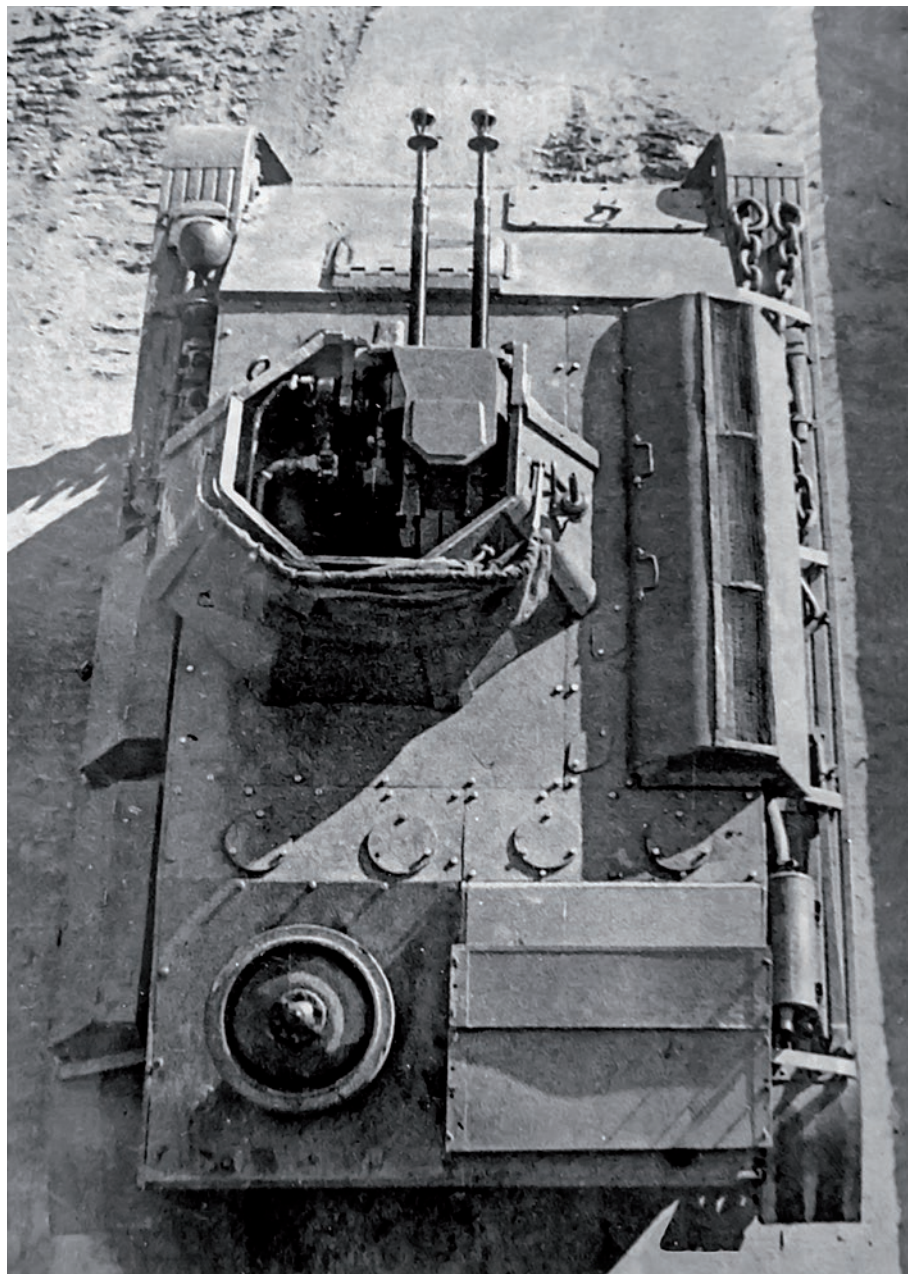
▲ Przeciwlotniczy T-90 w widoku od góry. Na tym zdjęciu dobrze widać, jak duże było przesunięcie karabinów w prawo i jak wyglądało opancerzenie przedniej części stanowiska. Przesunięcie broni zdecydowanie poprawiło warunki pracy strzelca. Z tyłu wieży znajduje się stelaż do rozpinania plandeki.
