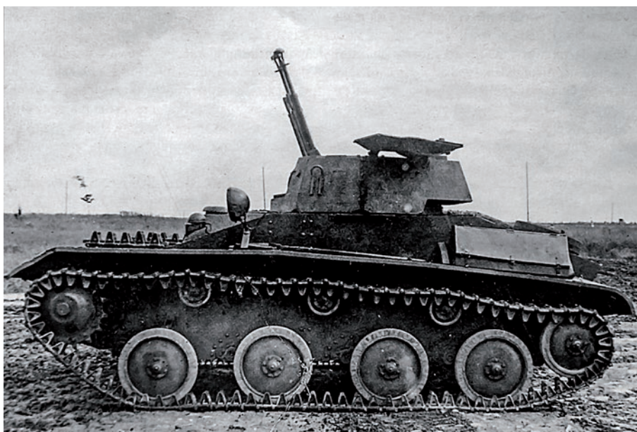
▲ Czołg przeciwlotniczy SZU był ostatnią próbą skonstruowania samobieżnego środka ochrony kolumn zmechanizowanych przed atakiem z powietrza i jednocześnie próbą wykorzystania bezwartościowych T-60. Tu pojazd demonstruje maksymalny kąt podniesienia luf. Panele pokrywają wieżę są w pełni odkryte.
