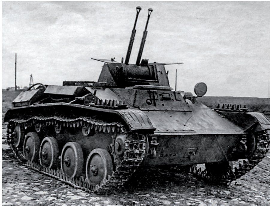
▲ Pojazd SZU w ujęciu ¾ od przodu na prawą burtę. Lufy karabinów DSzKT na maksymalnym kącie podniesienia. Sprawia to wrażenie, że wieża jest lekko skrzywiona w prawo. Klapy pokryw wieży są całkowicie otwarte. Z tyłu wieży widać gniazdo, do którego wkręcano antenę prętową.
