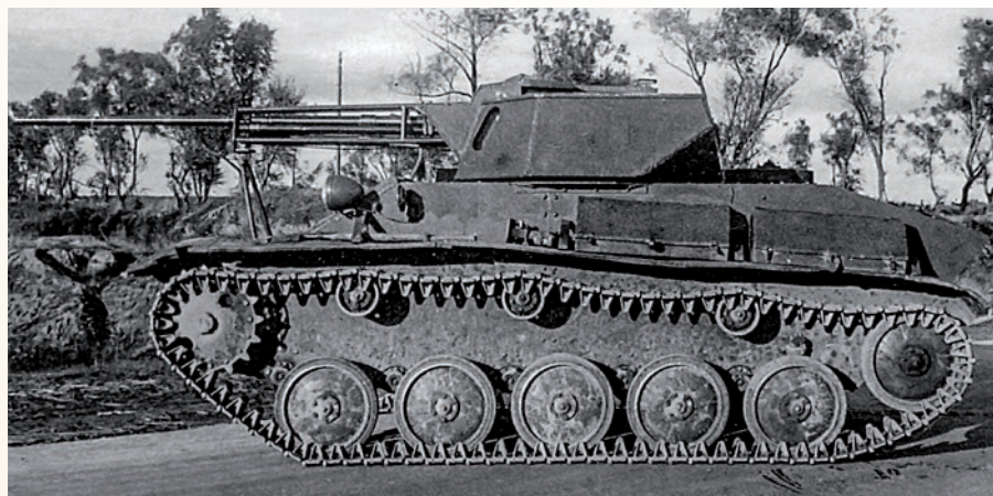
▲ Pojazd z OKB-15 zbudowany na bazie czołgu lekkiego T-70 w oficjalnej nomenklaturze był nazywany działem samobieżnym mimo, że był znacznie bliższy klasycznemu czołgowi. Na zdjęciu z sierpnia 1942 roku armata znajduje się w poziomym położeniu. Widać, że dla zmniejszenia masy podcięto tylne narożniki wieży.
