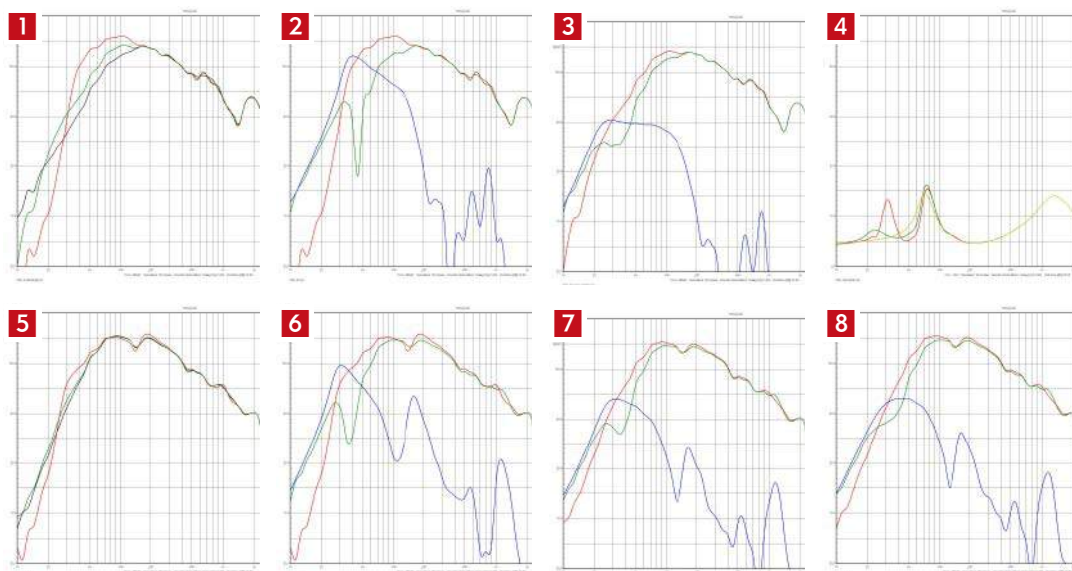
1. Charakterystyka w zakresie niskich częstotliwości Bronze 200 dla różnych strojeń bas-refleksu (i obudowy zamkniętej); 2. Charakterystyki składowe (głośniki/otwory) i wypadkowa Bronze 200 przy obydwu tunelach otwartych; 3. Charakterystyki składowe (głośniki/otwory) i wypadkowa Bronze 200 przy jednym tunelu zamkniętym; 4. Charakterystyka modułu impedancji Bronze 200 dla różnych strojeń bas-refleksu (i obudowy zamkniętej); 5. Charakterystyka w zakresie niskich częstotliwości LX5 mkII dla różnych strojeń bas-refleksu; 6. Charakterystyki składowe (głośniki/otwory) i wypadkowa LX5 mkII przy obydwu tunelach niewytłumionych; 7. Charakterystyki składowe (głośniki/otwory) i wypadkowa LX5 mkII przy jednym tunelu wytłumionym; 8. Charakterystyki składowe (głośniki/otwory) i wypadkowa LX5 mkII przy obydwu tunelach wytłumionych
