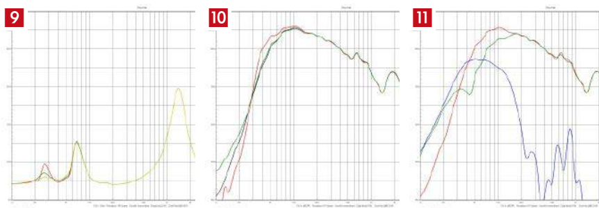
9. Charakterystyka modułu impedancji Bronze 200 dla różnych strojów bas-refleksu (i obudowy zamkniętej); 10. Charakterystyka w zakresie niskich częstotliwości Bronze 200 dla różnych strojów bas-refleksu za pomocą zatyczki z LX5 mkII; 11. Charakterystyki składowe (głośniki/otwory) i wypadkowa przy jednym tunelu wytłumionym Bronze 200 za pomocą zatyczki LX5 mkII
