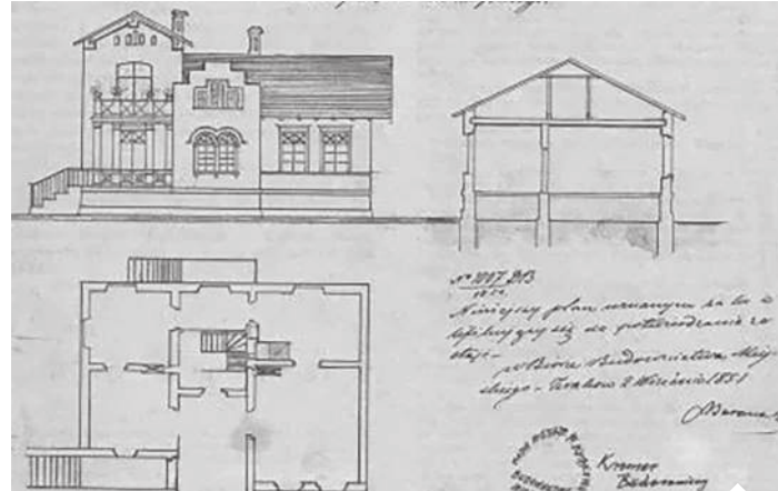
Projekt dworku Kossakówka autorstwa Karola Kremera bez późniejszych przybudówek | fot. arch./d
