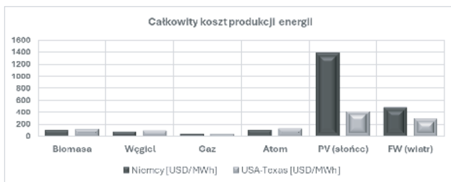
Rysunek 2. Całkowity koszt produkcji energii z różnych źródeł w Niemczech i USA
