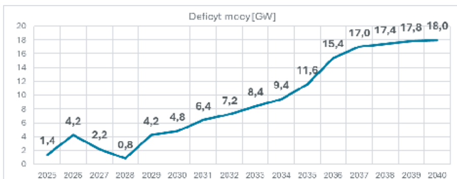
Rysunek 1. Prognozowany deficyt mocy w Polsce do 2040 r.
