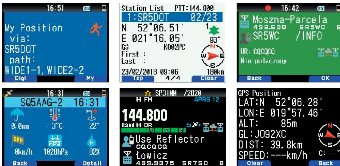
Rys. 10. Ekran TH-D74E przedstawiające różne tryby prezentacji danych: potwierdzenie przekazania przez digi SR5DOT pakietu APRS wysłanego z TH-D74, ekran z położeniem stacji SR5DOT oraz graficzna i liczbowa reprezentacja azymutu na podstawie danych APRS, informacja o przemienniku D-STAR SR5WC Moszna-Parcela, informacja o stacji pogodowej SQ5AAG-3 na podstawie radiowego pakietu APRS, ekran podczas łączności ze stacją SP3IMM przez reflektor D-STAR w Łowiczu, informacje o położeniu stacji rozmówcy zaprezentowane w systemie D-STAR
