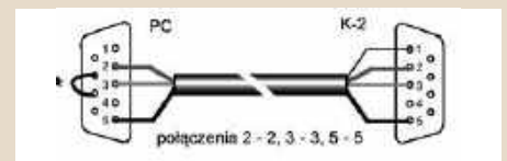
Kabel łączący PC z K-2
