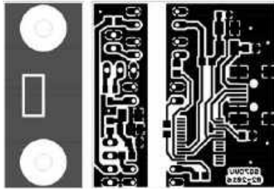
Rys. 2. PCB interfejsu CAT
