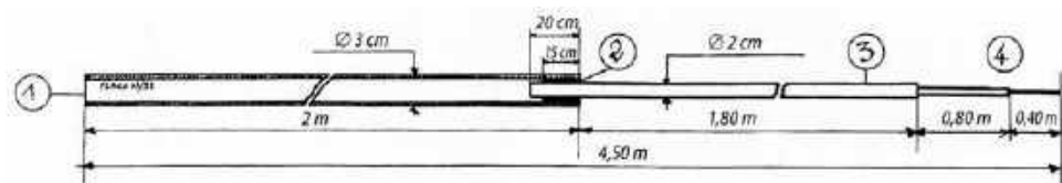
Rys. 4. Elementy promieniujące
