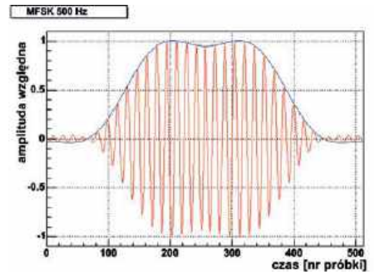
Rys. 7. Kształt impulsu
