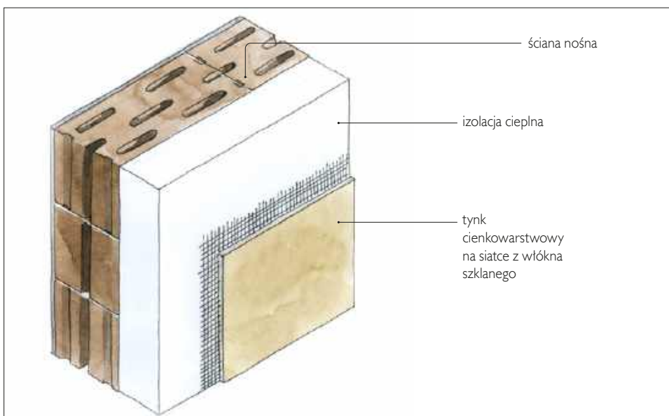
➊ Ocieplenie ścian metodą lekką moką, znaną także jako BSO lub ETICS polega na przyklejeniu izolacji do muru. Następnie pokrywa się ją warstwą kleju wzmocnionego siatką z włókna szklanego oraz tynkiem cienkowarstwowym.
