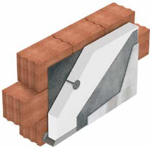
❶ Ściana dwuwarstwowa to zwykle mur nośny, styropian lub wełna mineralna oraz tynk cienkowarstwowy. CZAMANINEK
